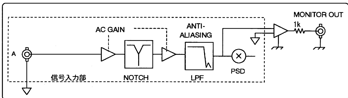
図4-6 入力からモニタ出力までの経路
