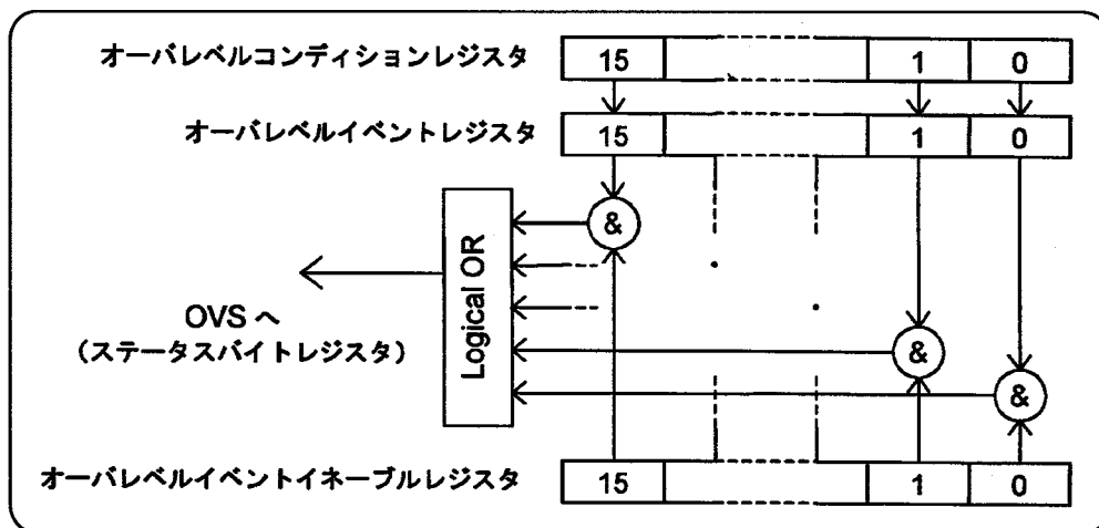
図5-7 オーバレベルステータス
