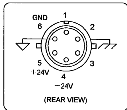
図3-3 ±24V電源出力
