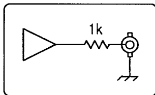
図3-7 DATA OUT、X OUT、Y OUT、MONITOR OUT出力回路
