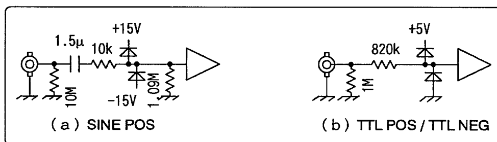
図3-5 REF IN入力回路
