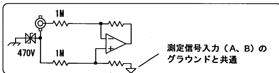
図3-4 AUX IN入力回路
