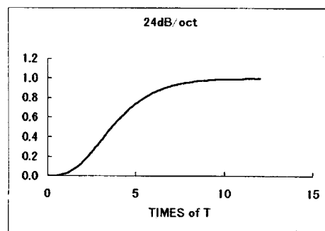
図4-5 ステップ応答波形
