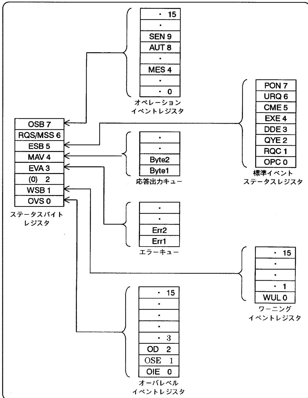
図5-3 ステータス構造図 (概要)
