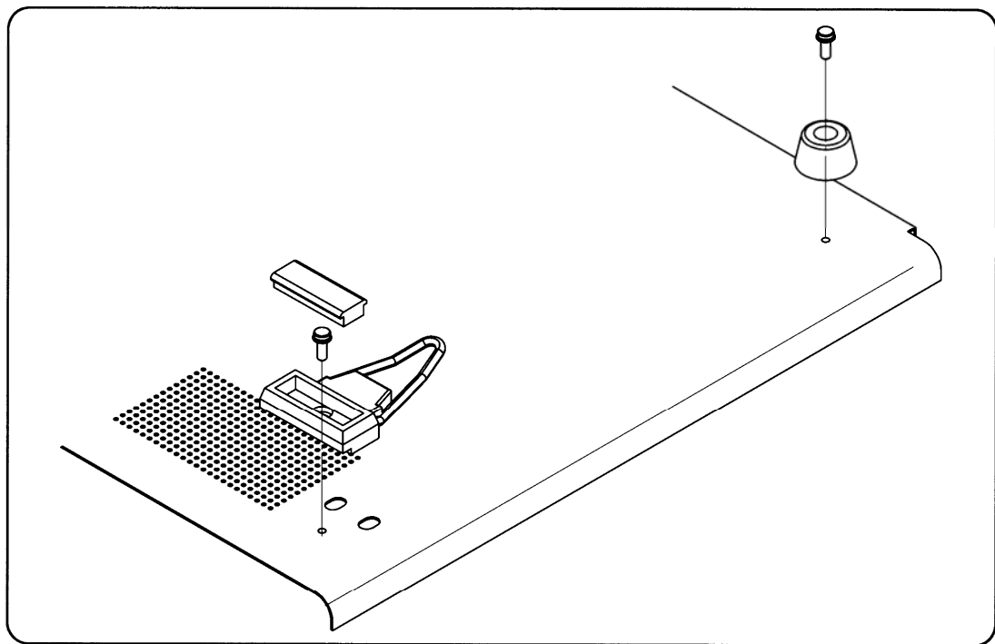
図2-3 フットの外し方
