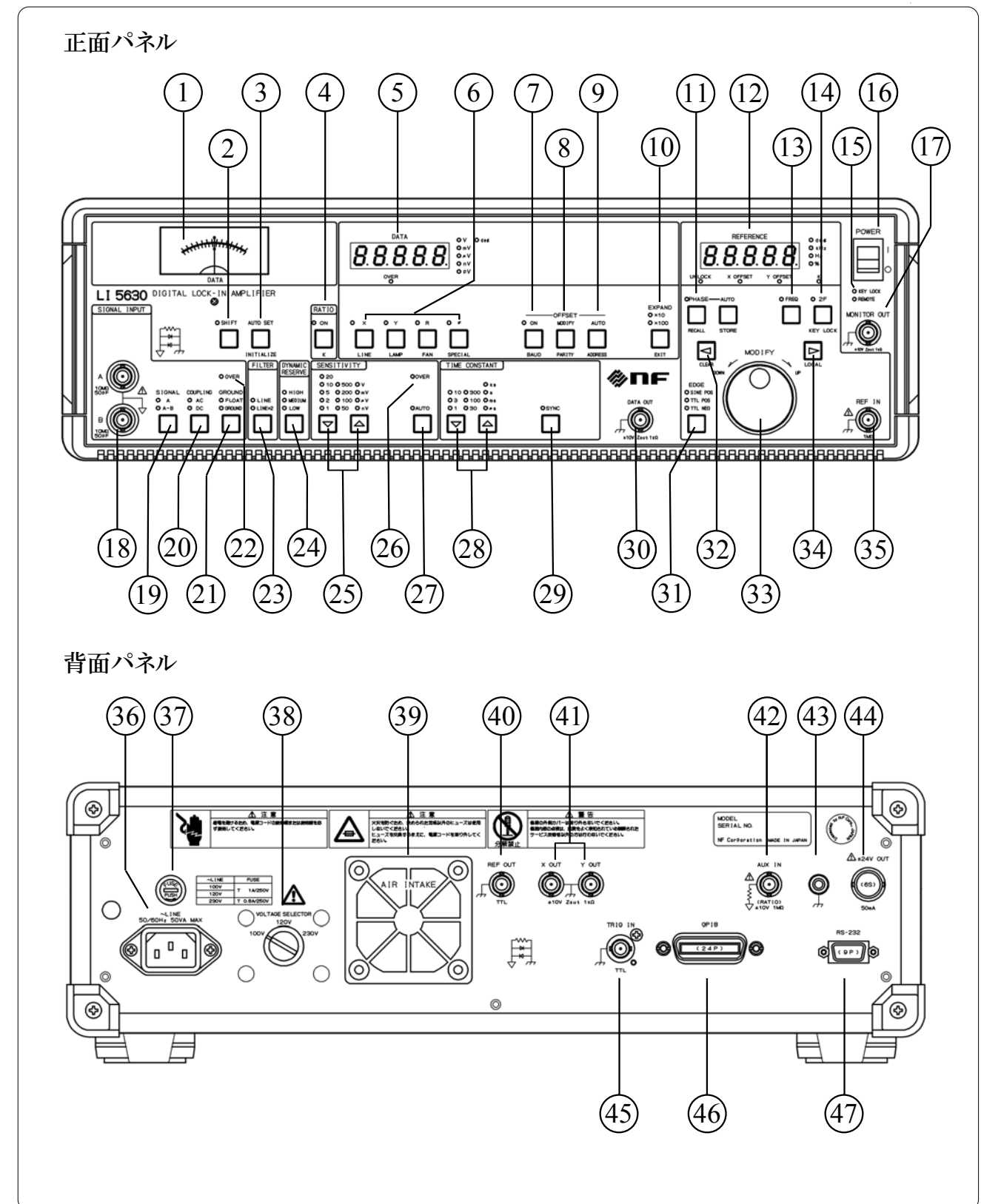
図3-1 正面・背面パネル図
