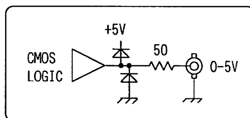
図3-6 REF OUT出力回路
