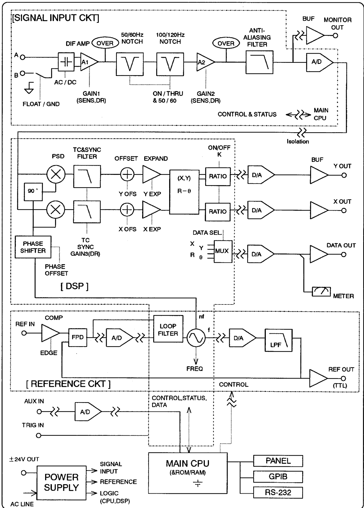
図 1-3 ブロック図
