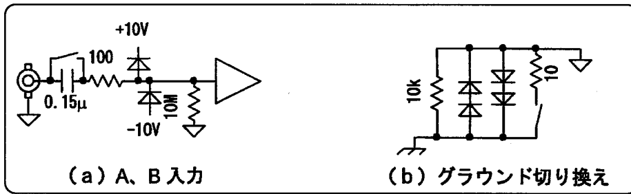
図3-2 SIGNAL INPUT (A、B) 入力回路とグラウンド
