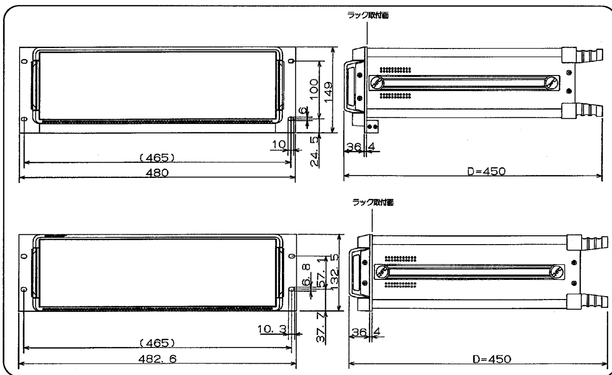
図2-1 LI5630 ラックマウント寸法図
