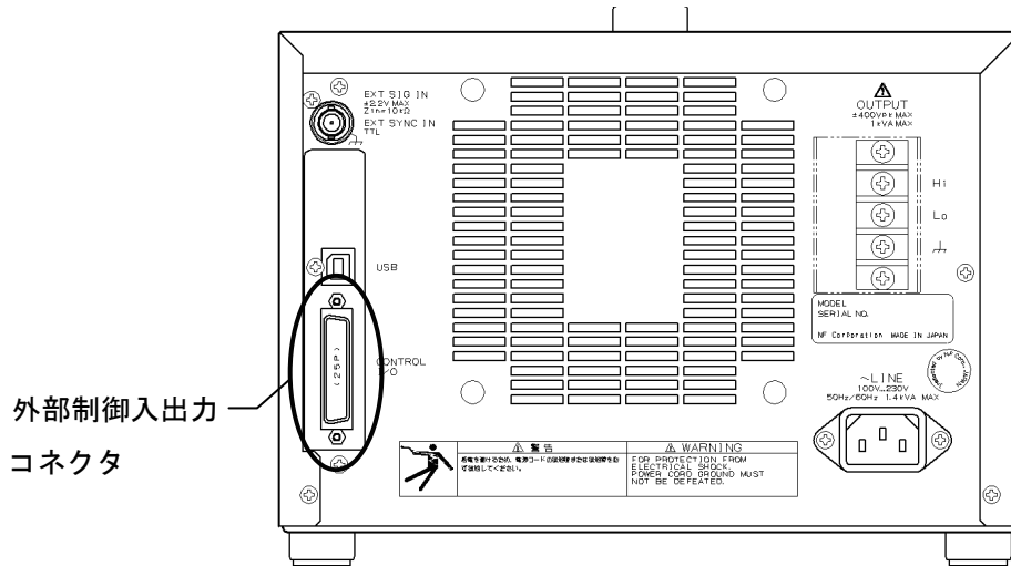
図 3-8 外部制御入出力コネクタ
