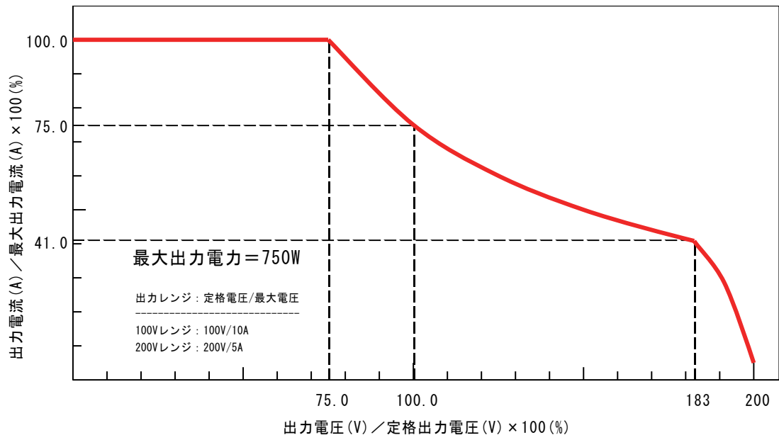
図 3-15 出力電圧 対 出力電流特性 (AC100V 入力, AC+DC-INT, AC=0)
