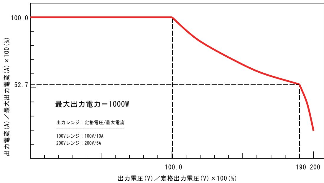
図 3-16 出力電圧 対 出力電流特性 (AC200V 入力, AC+DC-INT, AC=0)
