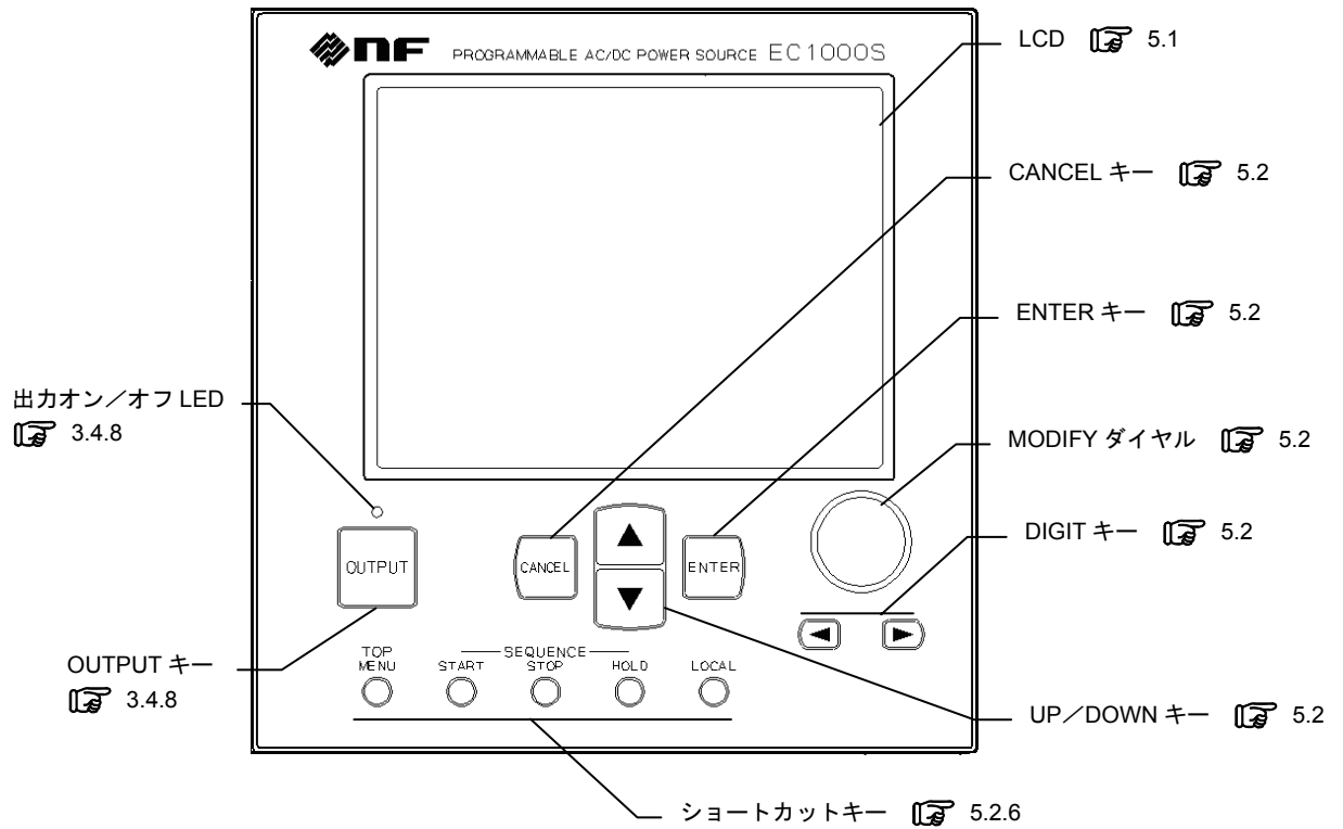
図 3-1 EC1000S 操作パネル
