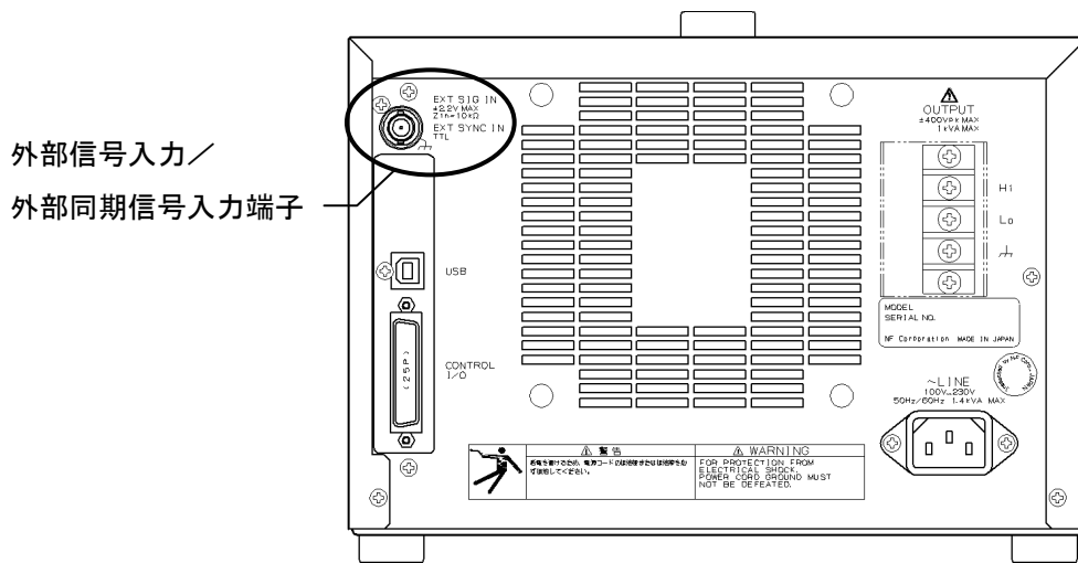
図 3-9 EXT SIG IN／EXT SYNC IN 端子
