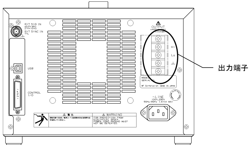
図 3-5 出力端子（リア）
