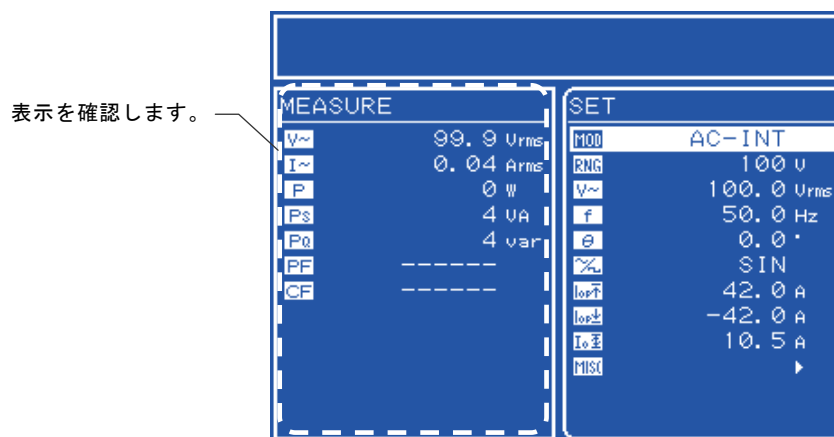
図 2-3 動作確認
