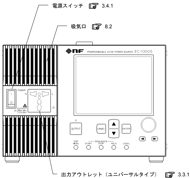
図 3-2 EC1000S フロントパネル
