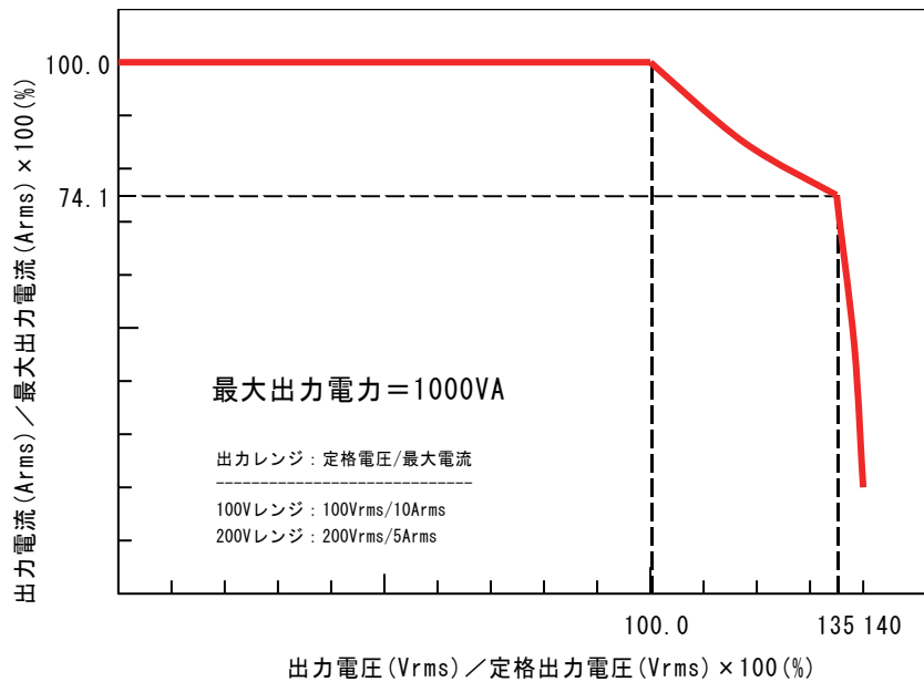
図 3-14 出力電圧 対 出力電流特性（AC200 V 入力，AC-INT）
