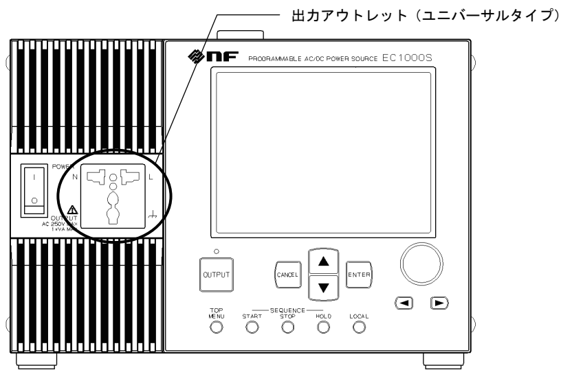
図 3-4 出力アウトレット（フロント）
