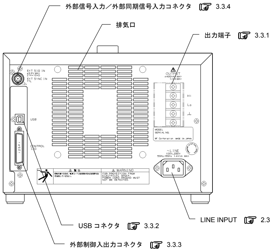
図 3-3 EC1000S リアパネル
