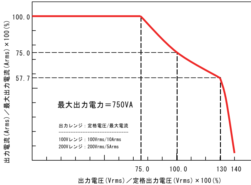
図 3-13 出力電圧 対 出力電流特性（AC100 V 入力，AC-INT）
