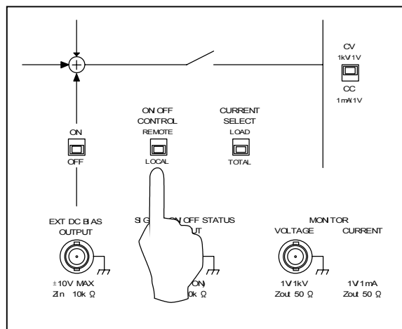
Figure4-22. Local settings
