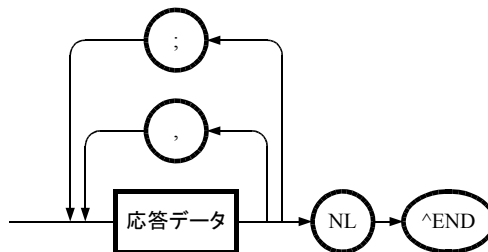
図 3.14 応答メッセージのシンタックス
