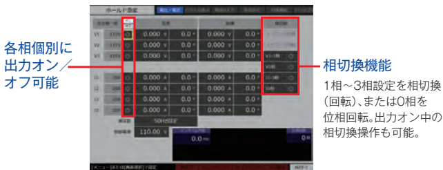
従来機種による 電圧4相・電流4相システム (自動試験ソフトウェア付システム)
