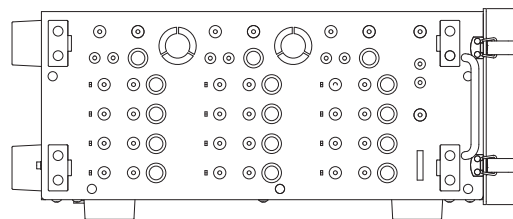
左側面図 (端子保護カバーなし)
