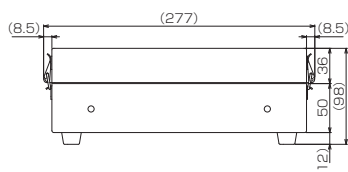
カバーなし
