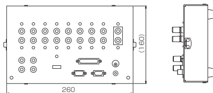
カバーなし
