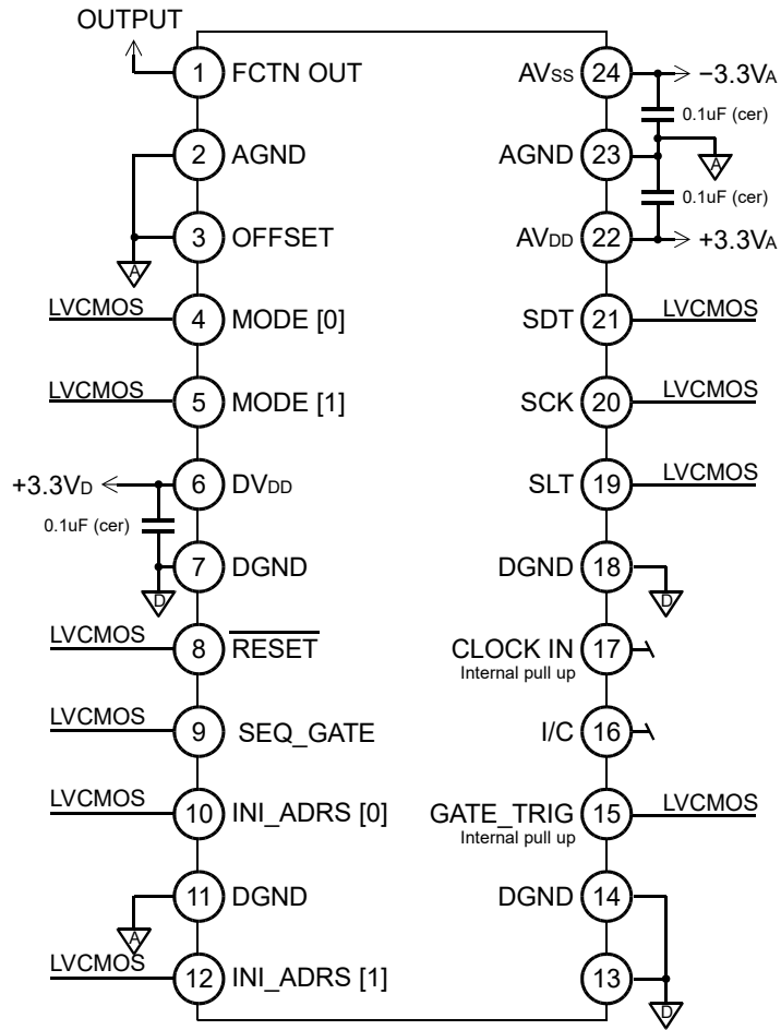
図 2 基本接続図（正負両電源使用）
