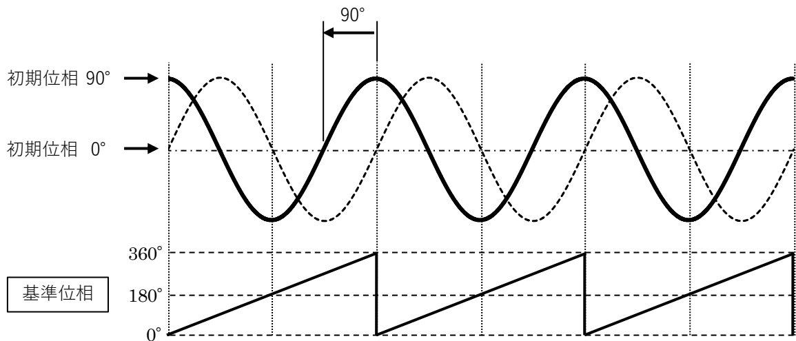
図 10 初期位相設定 0^\circ と 90^\circ の正弦波比較
