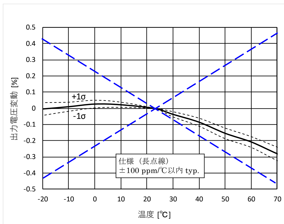
図 19 出力電圧変動対温度特性
