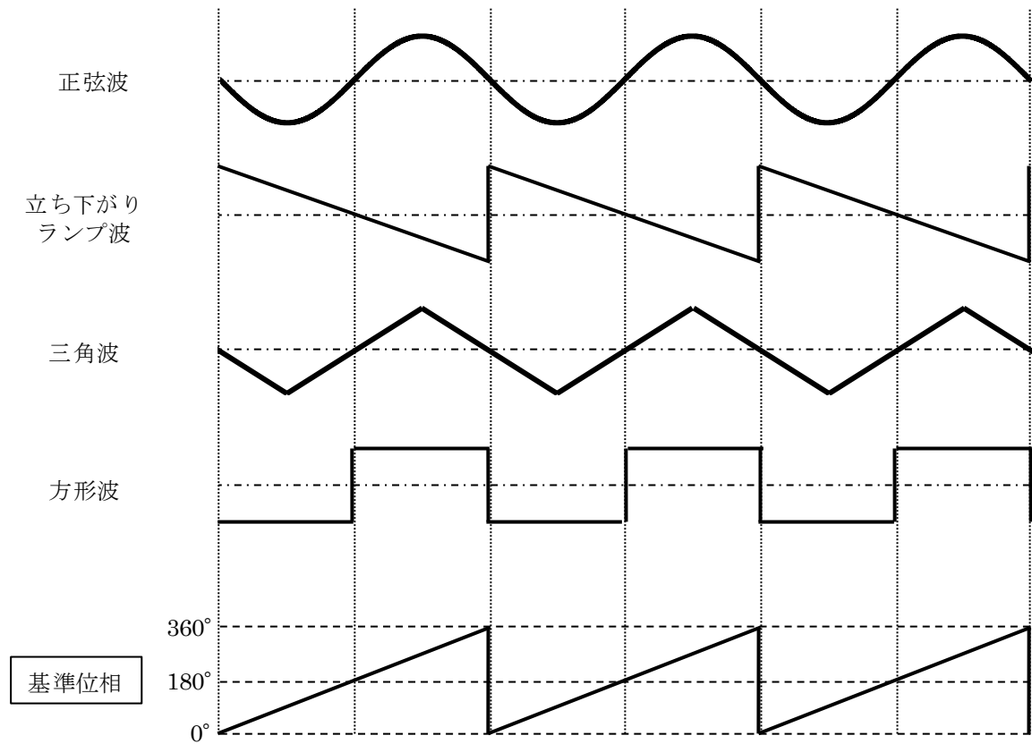
図 9 基準位相と各波形の関係 (初期位相 0°, 振幅 -1.0, オフセット 0.0)
