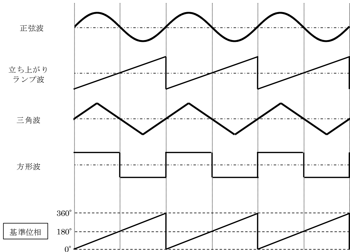
図 11 波形タイムチャート
