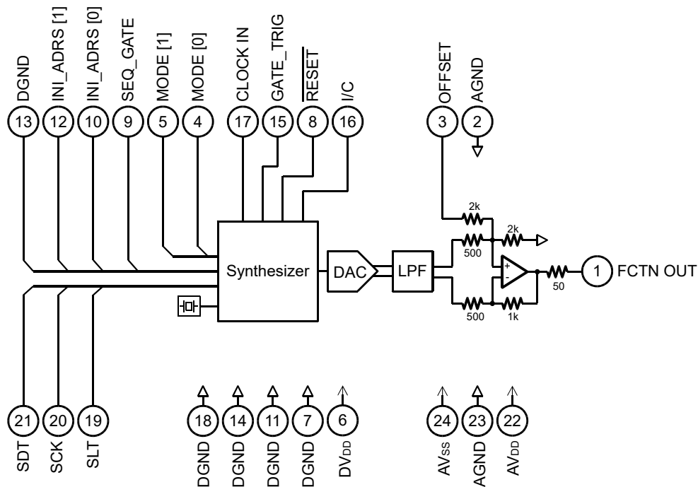
図 1 ブロック図
