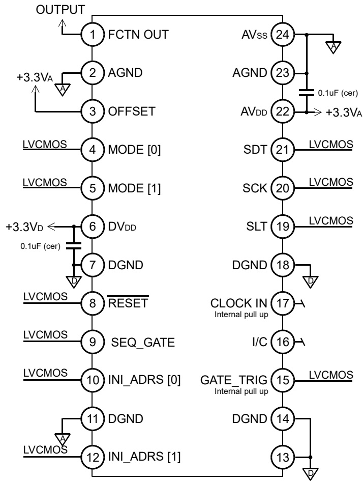
図 3 基本接続図 (片電源使用)
