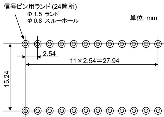
図 15 パターン寸法図
