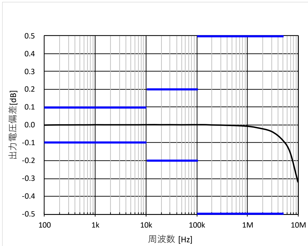
図 20 出力電圧偏差対周波数特性
