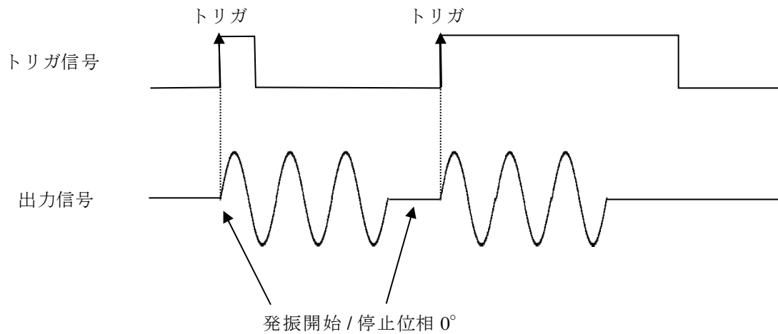
図 5 トリガ発振時 (3 周期発振設定の場合)
