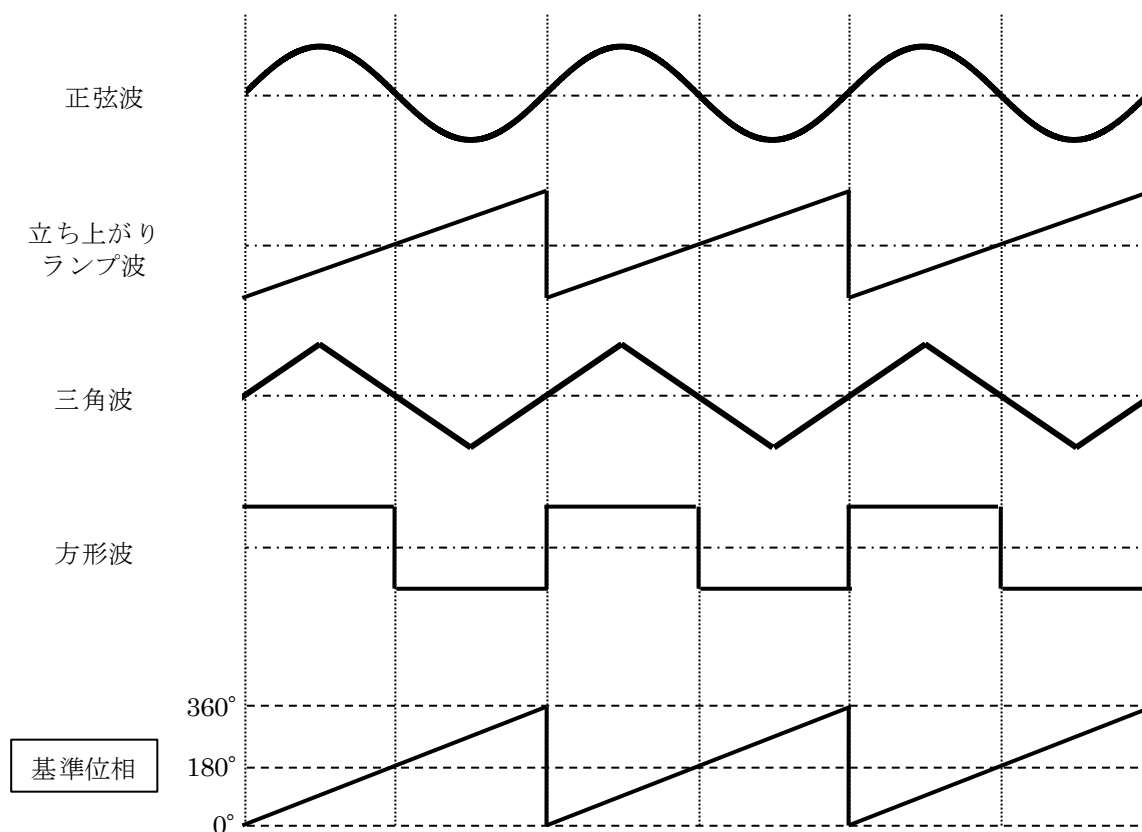
図 8 基準位相と各波形の関係 (初期位相 0^\circ 、振幅 +1.0 、オフセット 0.0 )
