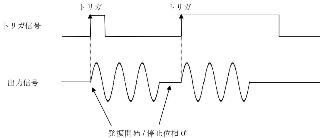
図 13 トリガ発振時
