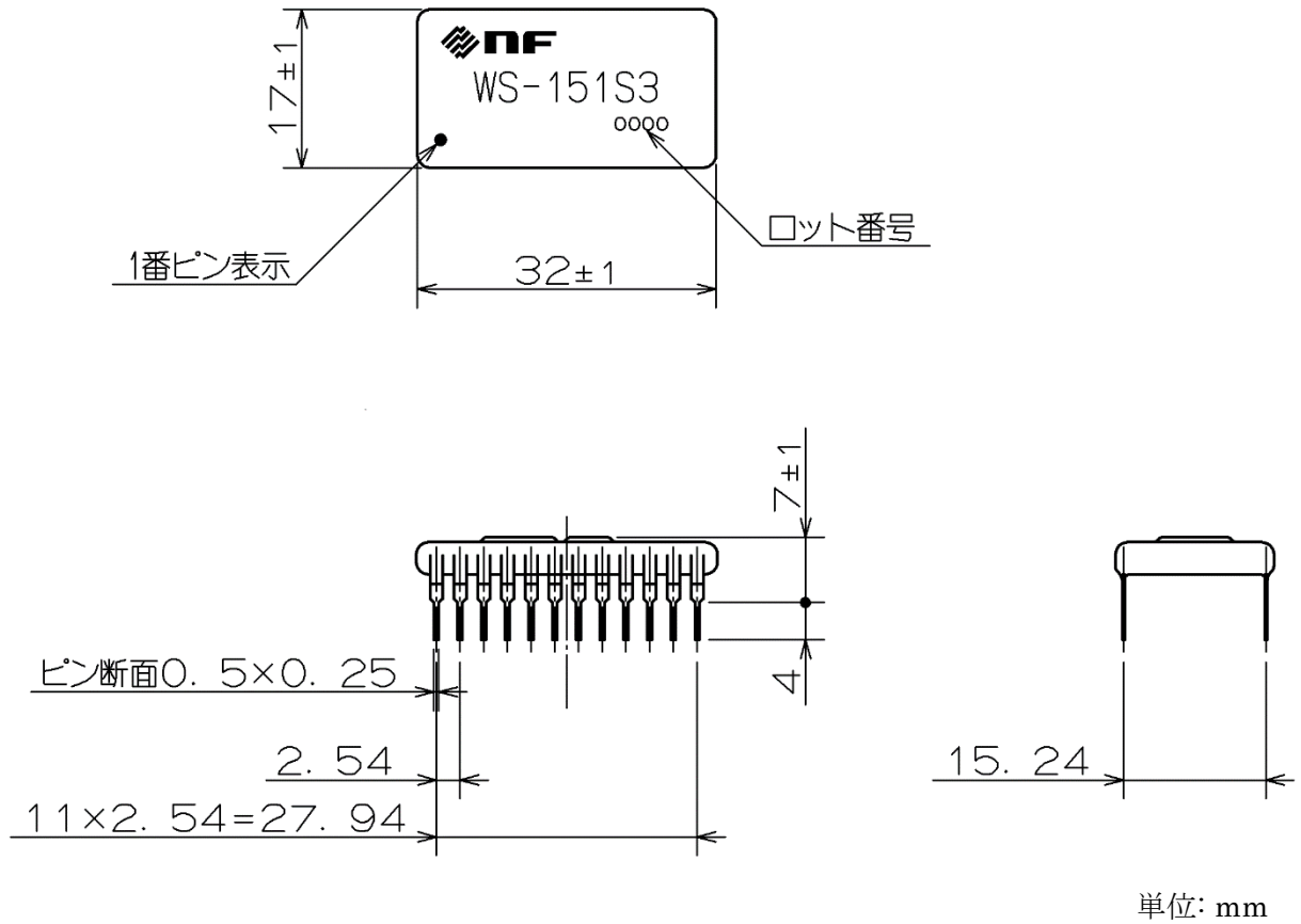
図 14 モジュール外観寸法
