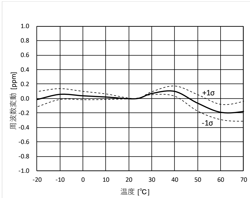
図 18 出力周波数変動対温度特性
