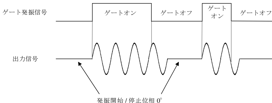
図 1 ゲートと発振の開始・停止の関係
