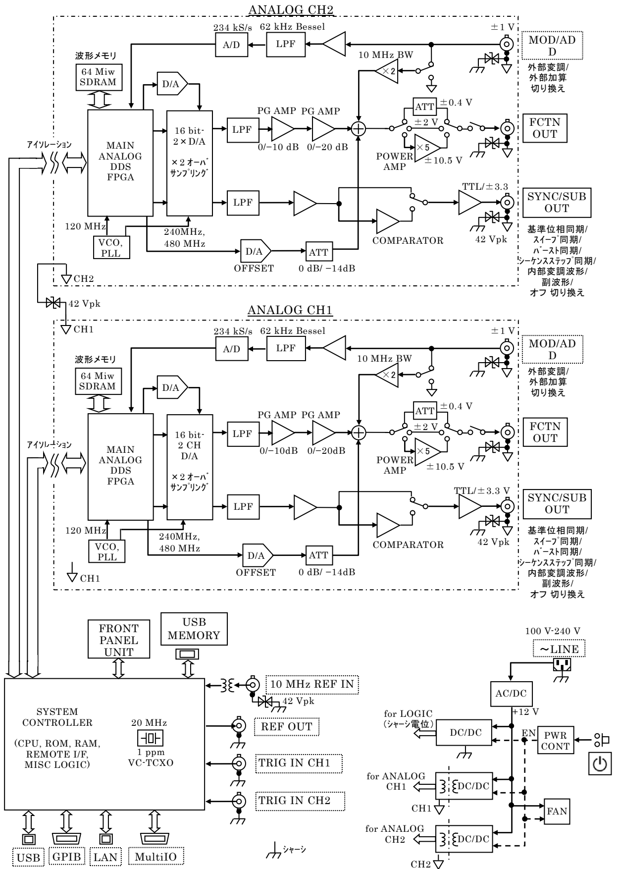
図 1-2 WF1984 ブロック図
