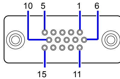
図 3-5 マルチ入出力コネクタ ピン配置図
