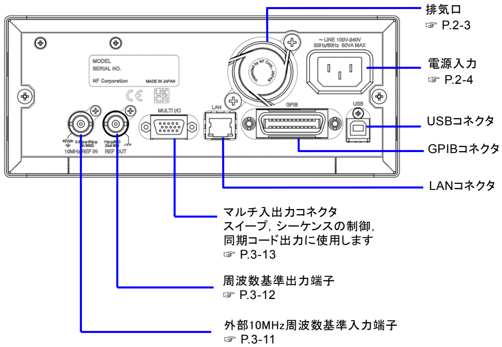
図 3-2 WF1983 背面パネル
