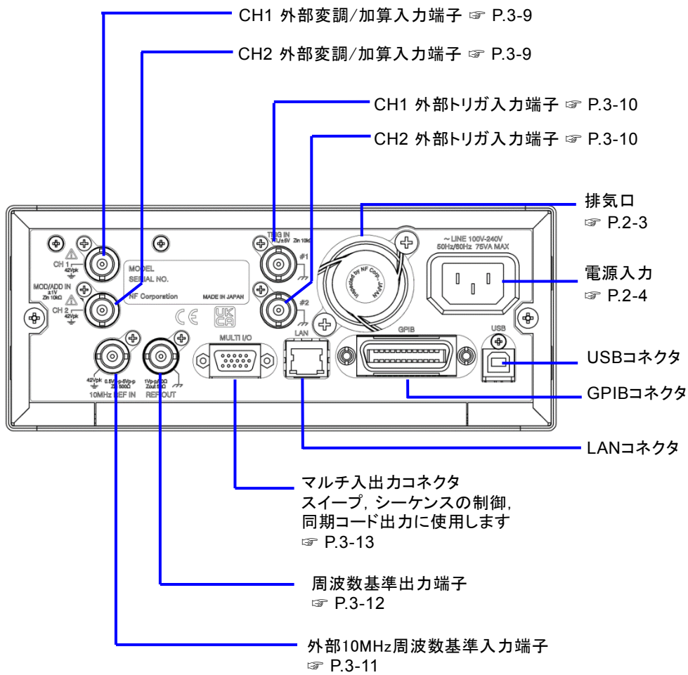
図 3-4 WF1984 背面パネル
