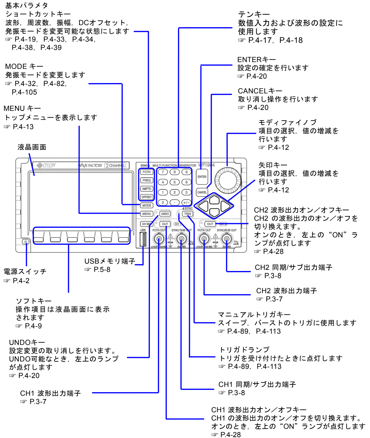
図 3-3 WF1984 正面パネル
