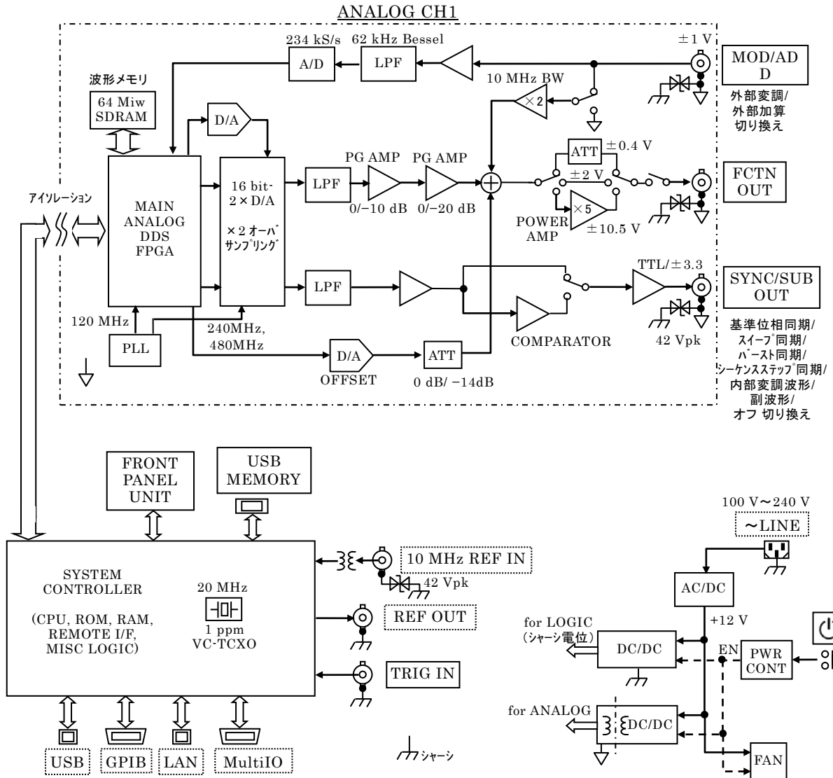
図 1-1 WF1983 ブロック図
