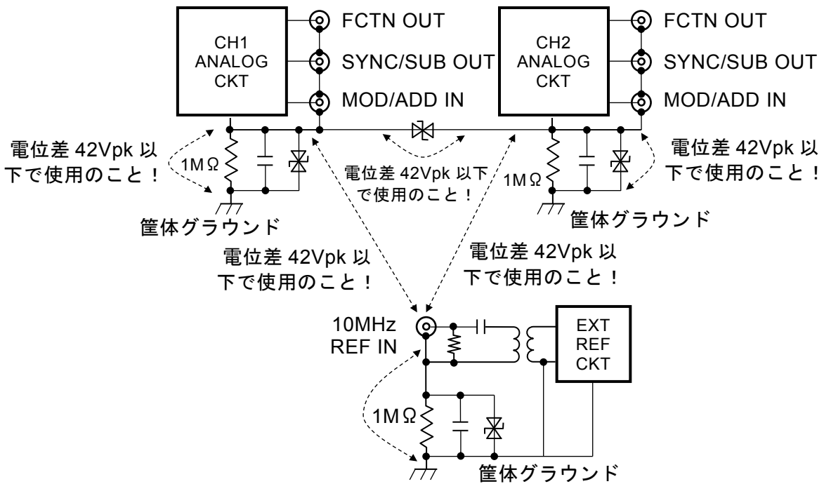
図 3-7 WF1984 のフローティンググラウンド接続時の注意
