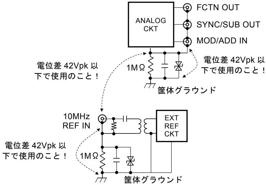
図 3-6 WF1983 のフローティンググラウンド接続時の注意
