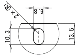
A 部詳細 (1 : 1)
