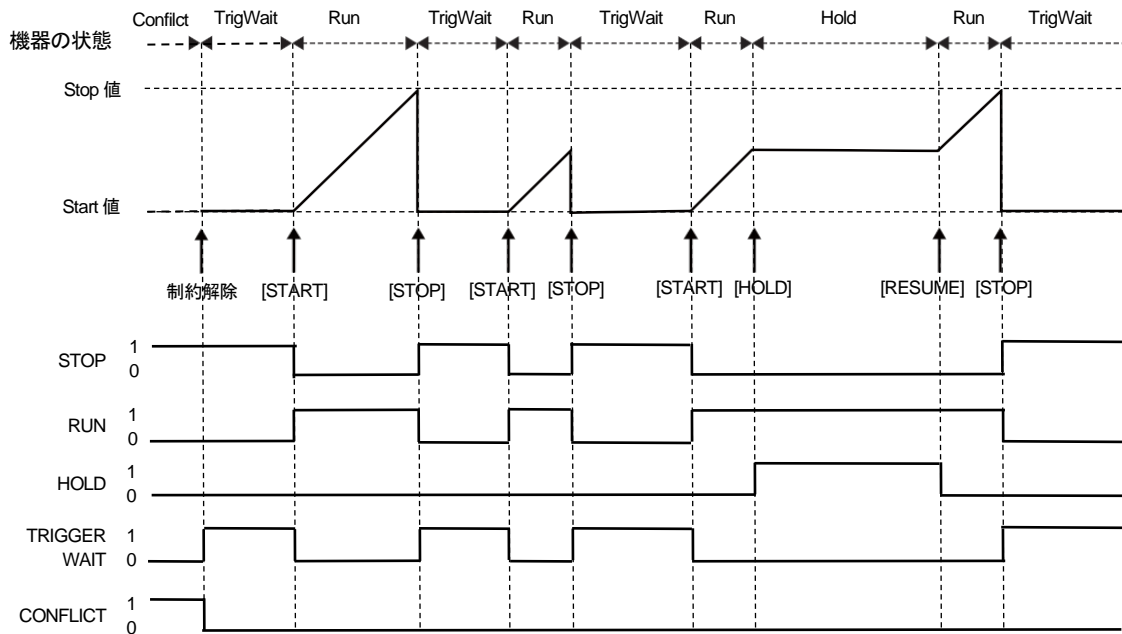
図 3.6 単発スイープ、ゲーテッド単発スイープ時の出力とオペレーション・ステータス・レジスタ (ビット 7-11) の関係
