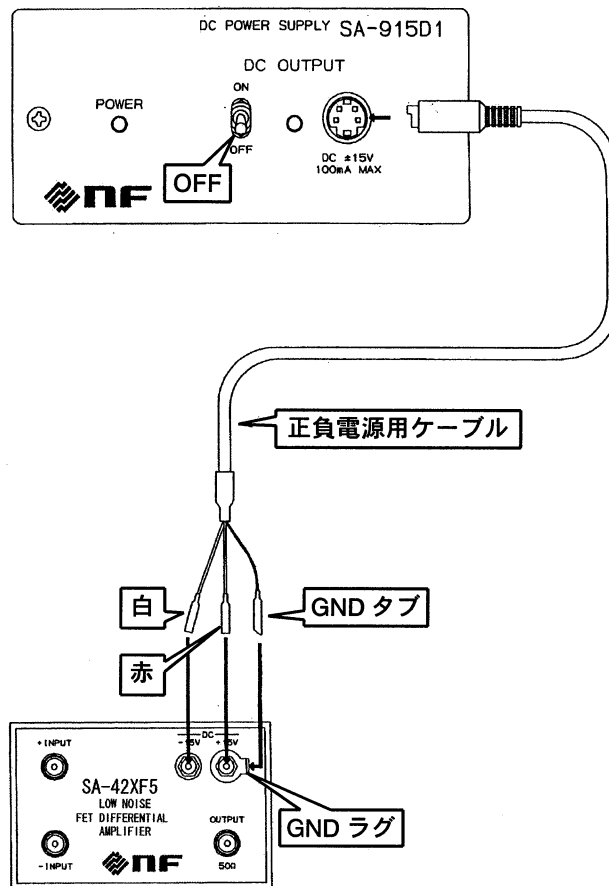
図 2-1 専用電源との接続
