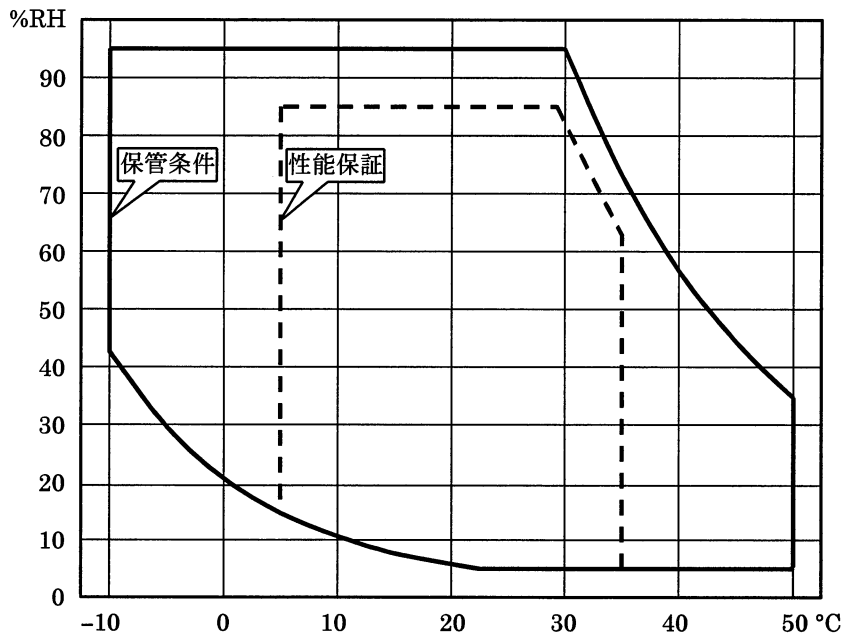
図 5-1 温湿度範囲説明図
