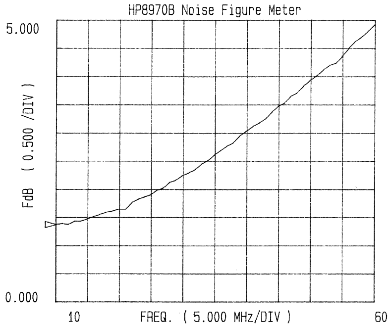
図 6-2 雑音指数周波数特性 10 MHz~60 MHz
