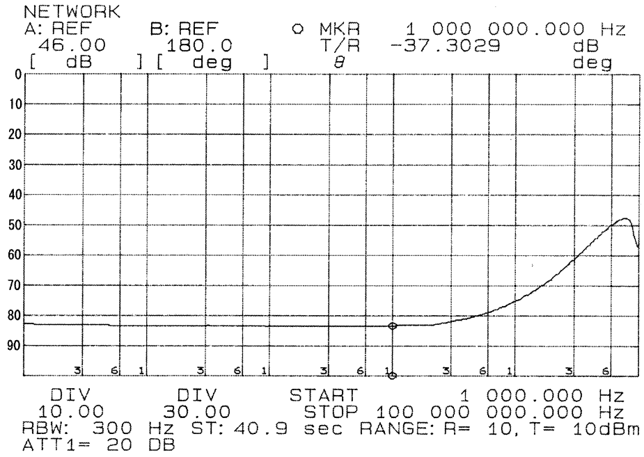
图 6-6 同相入力電圧除去比周波数特性 1 kHz~100 MHz
