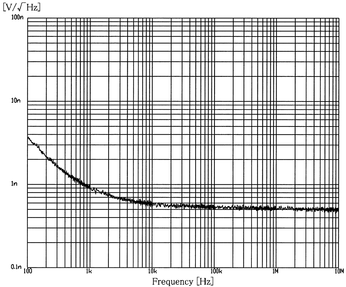
図 6-1 入力換算雑音電圧密度 100 Hz～10 MHz
