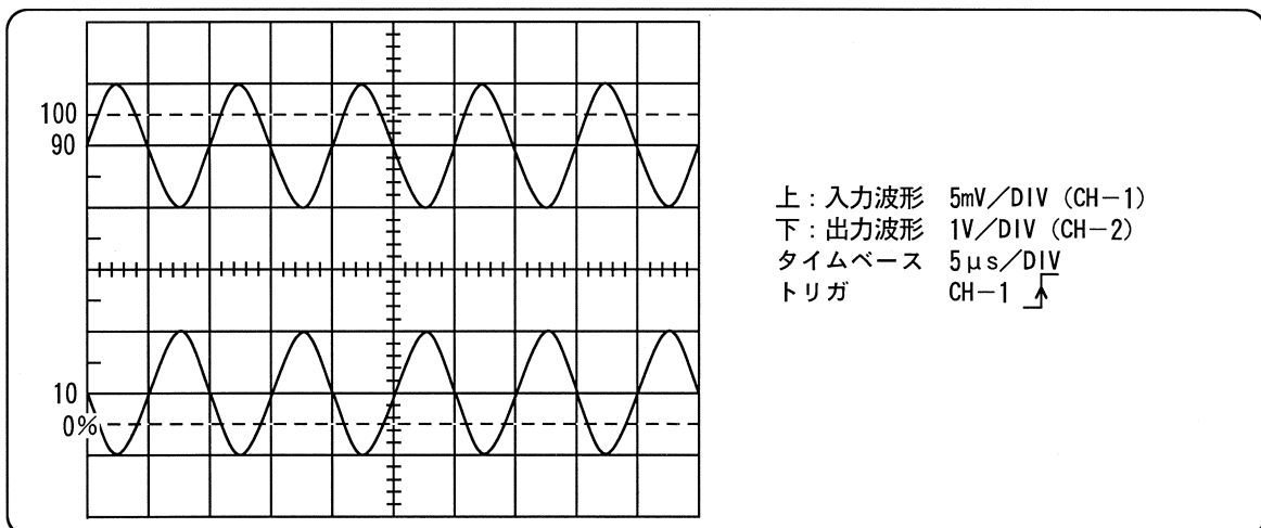
図5-2 入出力波形
