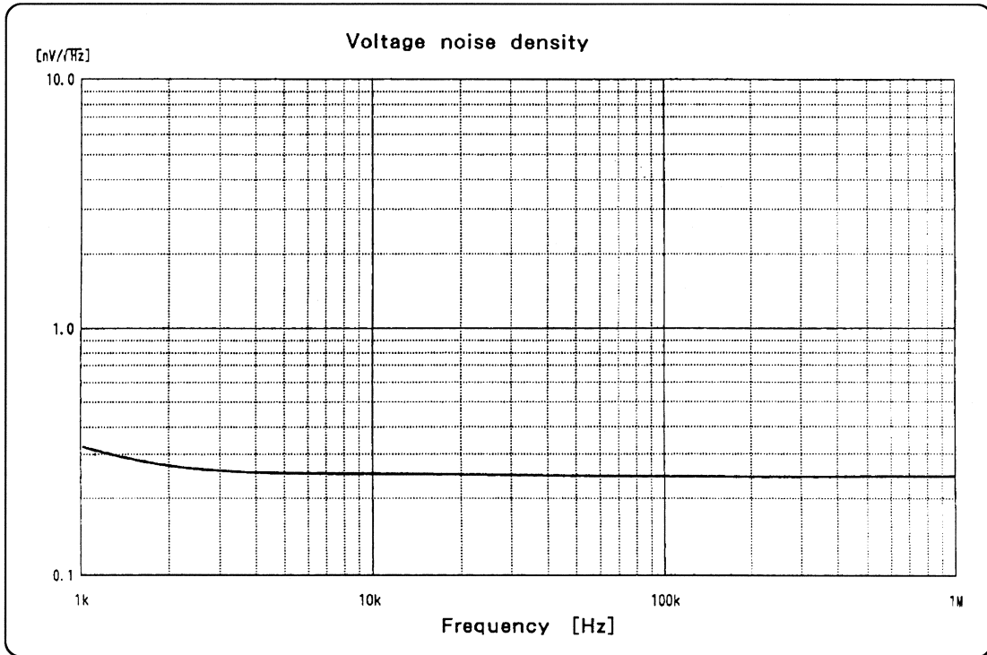
図6-1 入力換算雑音電圧密度 1kHz~1MHz
