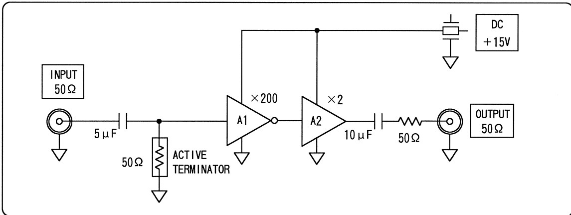
図4-1 ブロックダイアグラム
