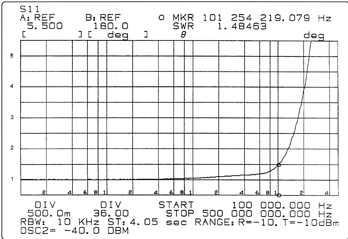
図6-5 入力VSWR周波数特性 100kHz~500MHz
