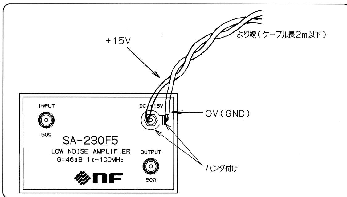
図 3-2 SA-915D1 以外の電源との接続
