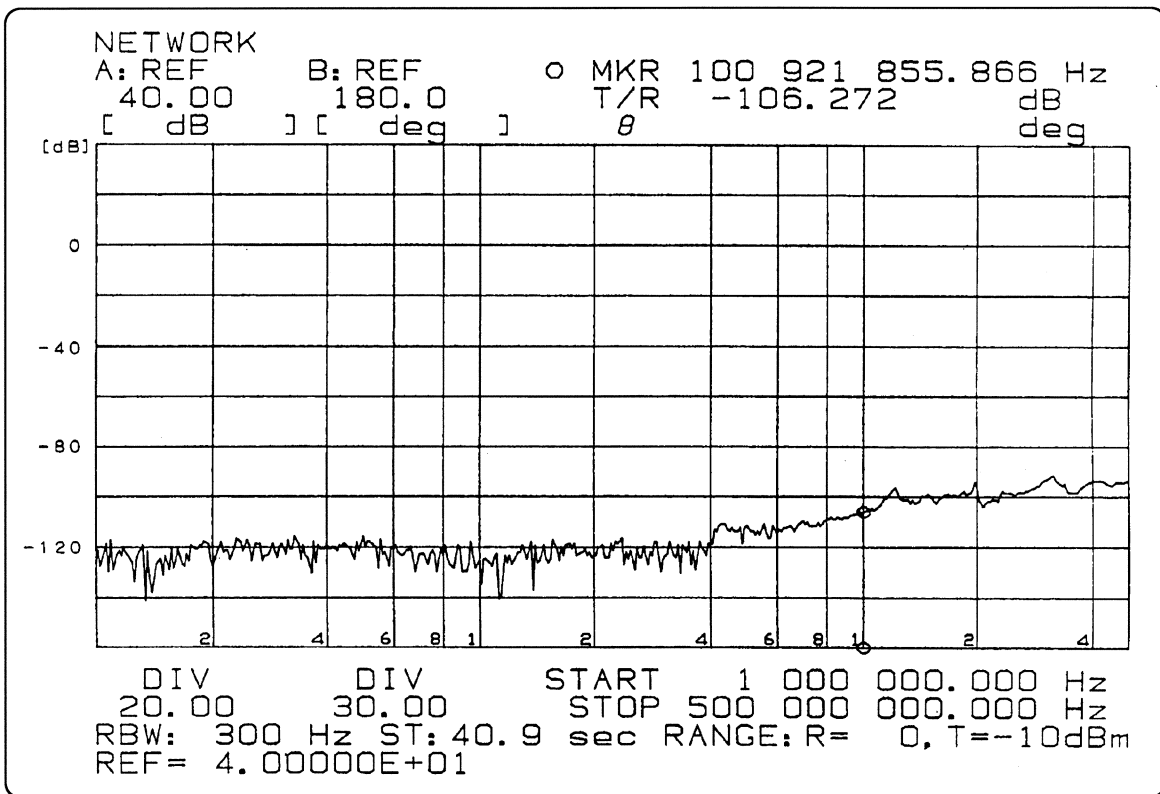
図6-7 逆方向伝達利得周波数特性 1MHz~500MHz
