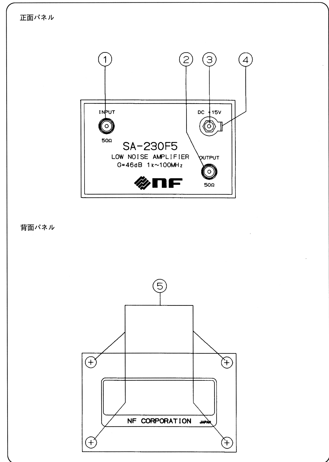
図3-3 正面・背面パネル図
