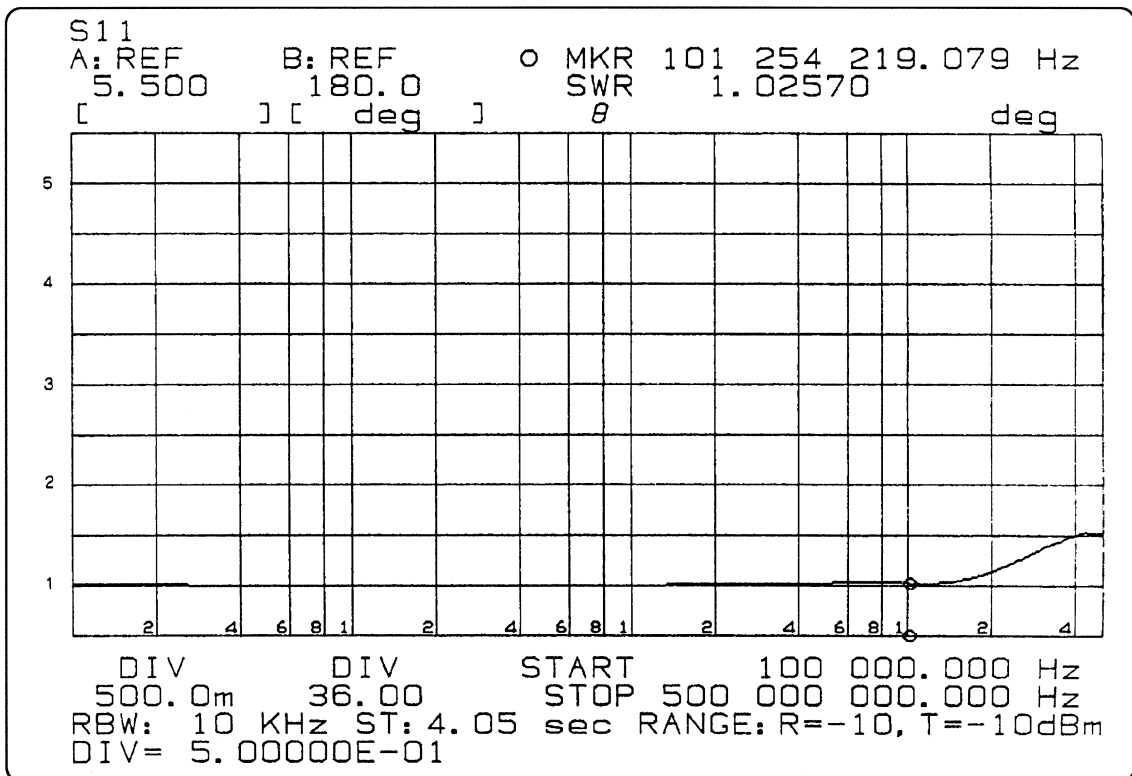
図6-6 出力VSWR周波数特性 100kHz~500MHz
