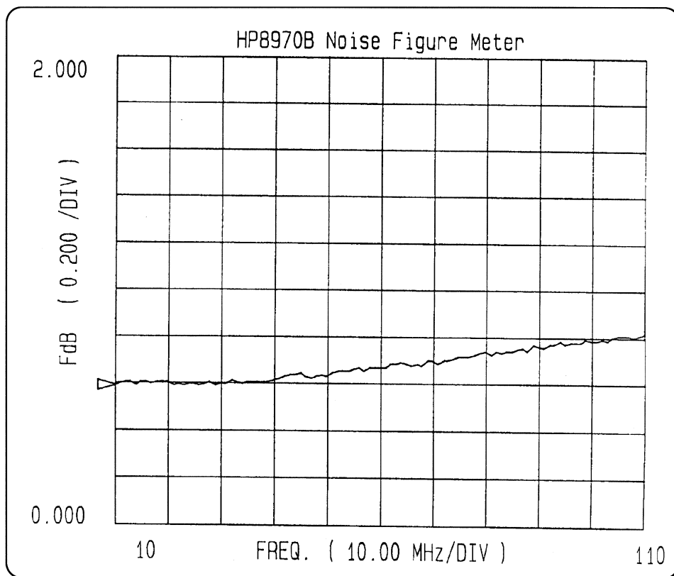
図6-2 雑音指数周波数特性 10MHz~110MHz
