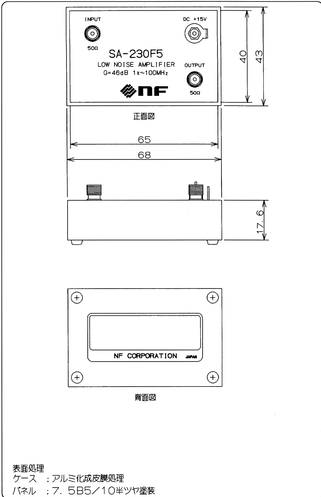
図1-1 外形寸法図
