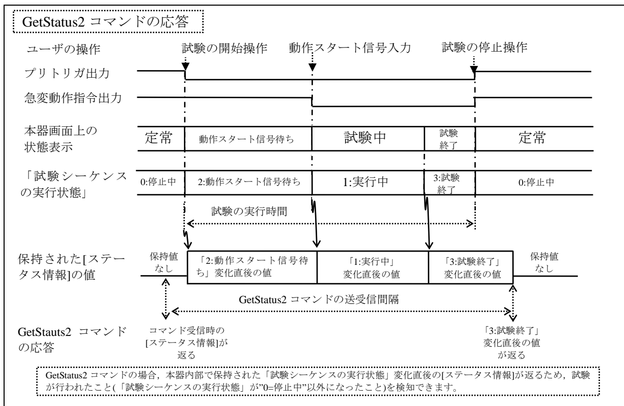
図 1-2 GetStatus コマンドと GetStatus2 コマンドの差異
