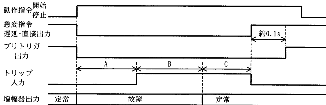
図 3-19 動作・復帰同時計測モードの動作
