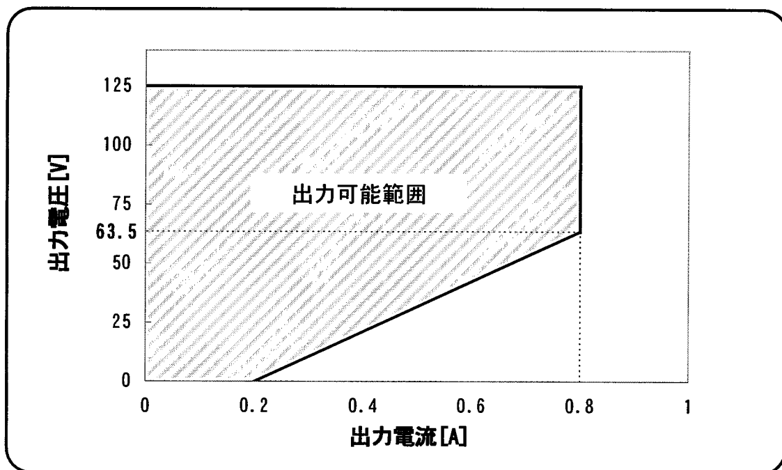
図 9-1 電圧出力 125V レンジ出力電流特性
