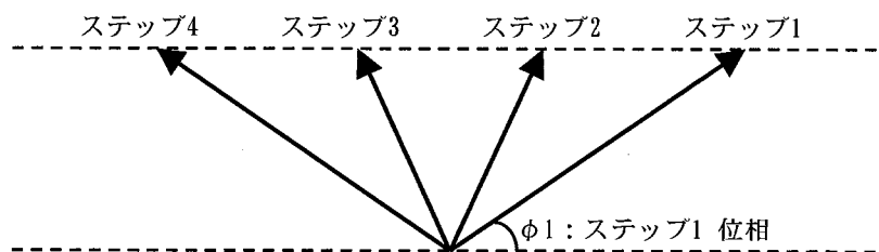
図 3-23 SOR 試験モードの各ステップの設定例(ベクトル図)
