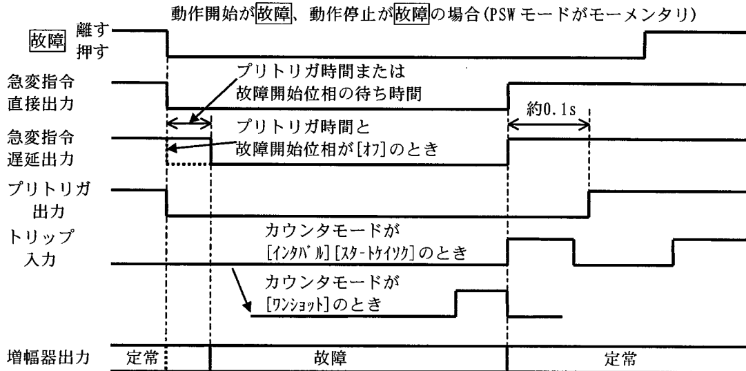
図 3-11 ホールド急変の動作、自動復帰[お]
