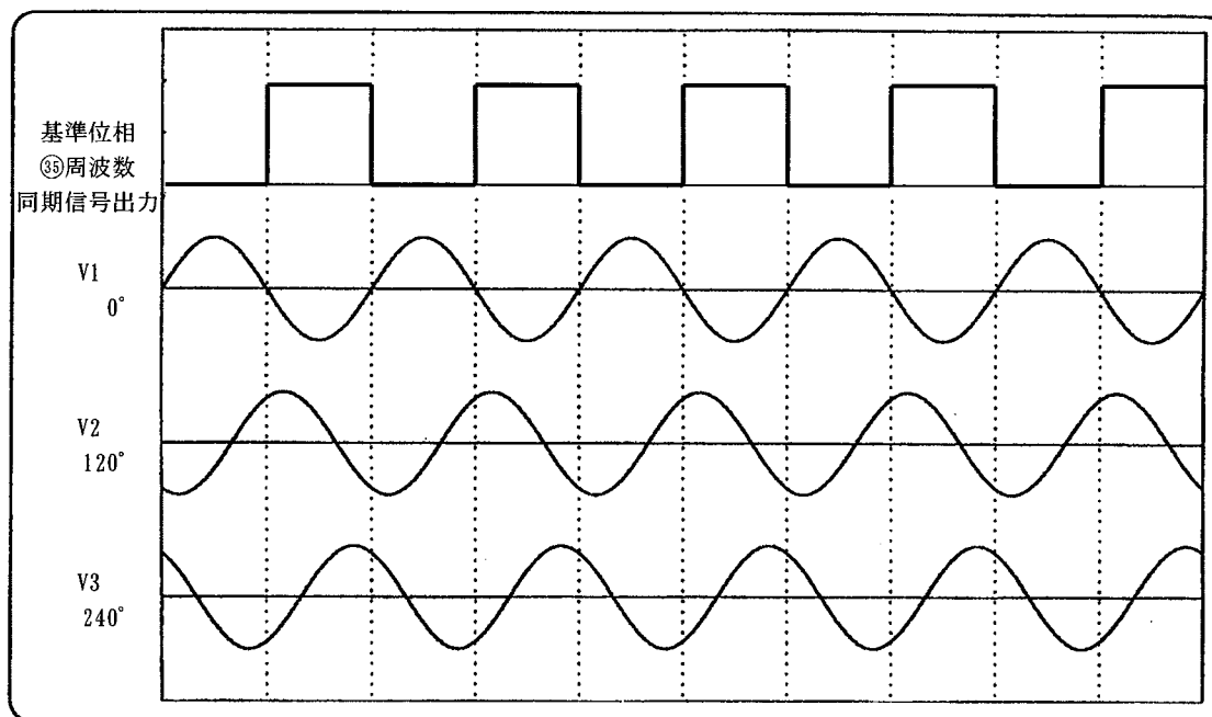
図 3-6 V1: 0^\circ 、V2: 120^\circ 、V3: 240^\circ の出力波形
