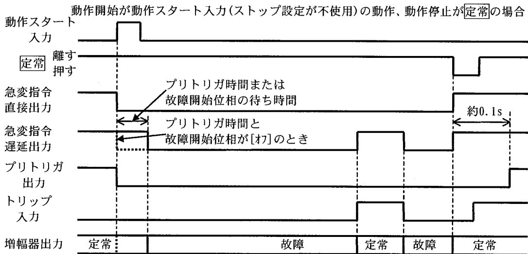
図 3-13 ノンホールド急変の動作
