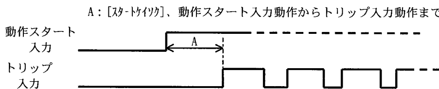
図 3-15 スタート計測の計測内容
