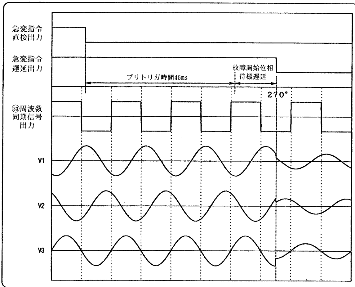
図 3-18 プリトリガ時間と故障開始位相[オ]の急変開始タイミング例
