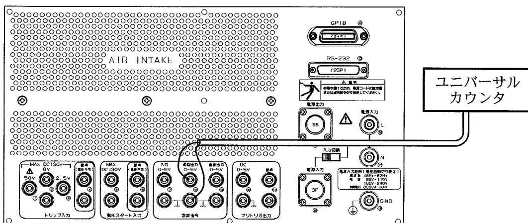
図 8-4 ユニバーサルカウンタの接続(カウンタ確度)
