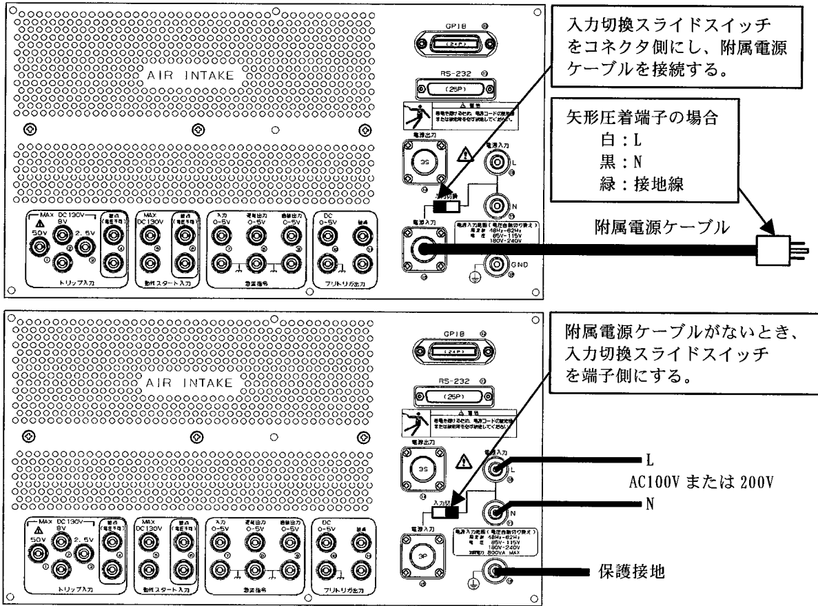
図 2-2 電源ケーブルの接続
