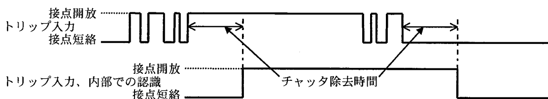
図 3-10 チャッタ除去機能の動作
