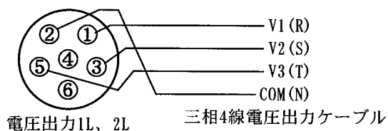
図 3-1 電圧出力 1L、2L コネクタと三相 4 線電圧出力ケーブルのピン接続
