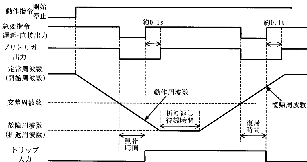
図 3-22 95 試験モードの動作
