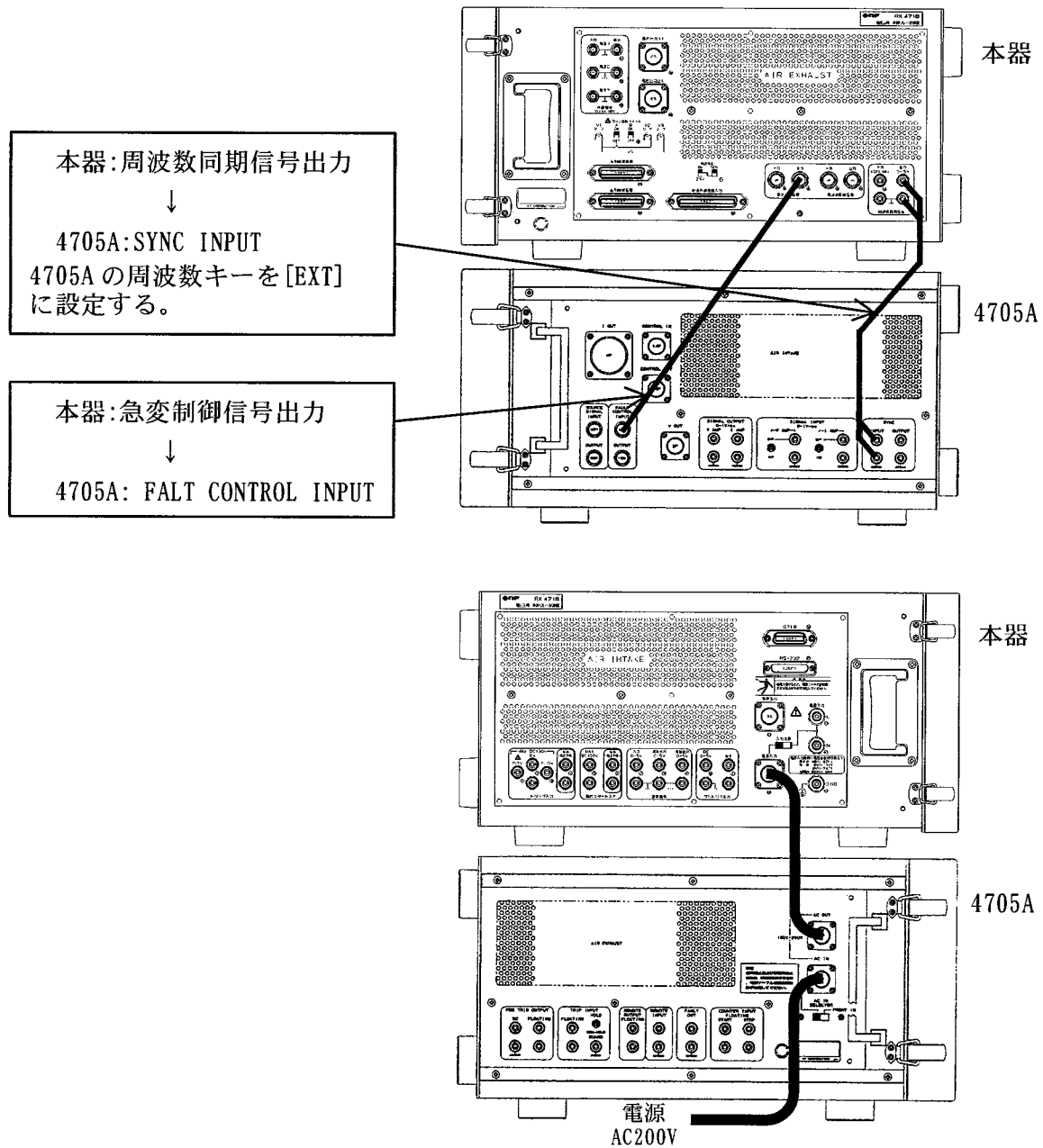
図 4-8 4705A 同時故障急変の接続
