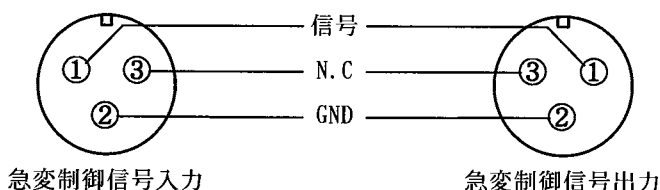
図 4-5 急変制御信号入出力(TPR-33用)のピン接続
