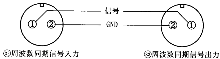
図 4-4 周波数同期信号入出力(TPR-33用)のピン接続
