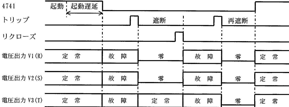
図 4-3 遮断相選択機能の動作例
