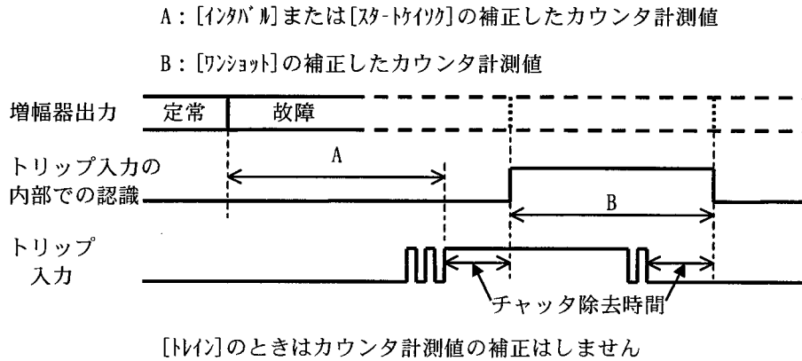
図 3-16 トリップ入力チャッタ除去機能[オ]のときのカウンタ計測値
