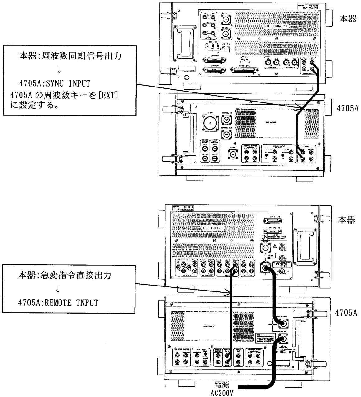
図 4-6 4705A プリトリガ時間、故障開始位相を個別設定の接続
