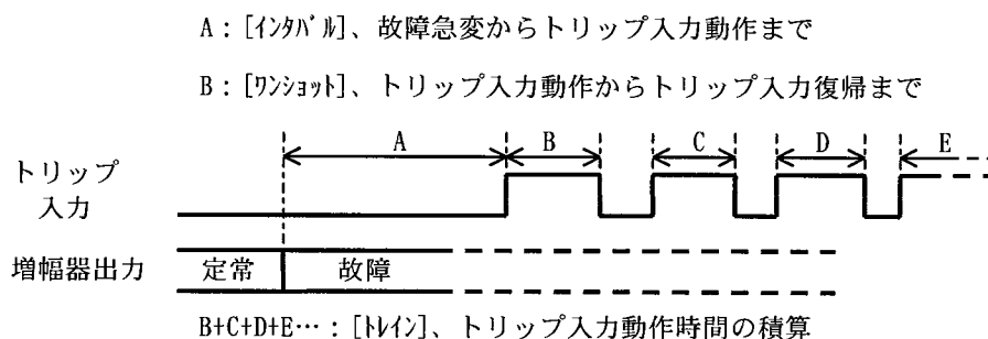
図 3-14 インタバル、ワンショット、トレインの計測内容
