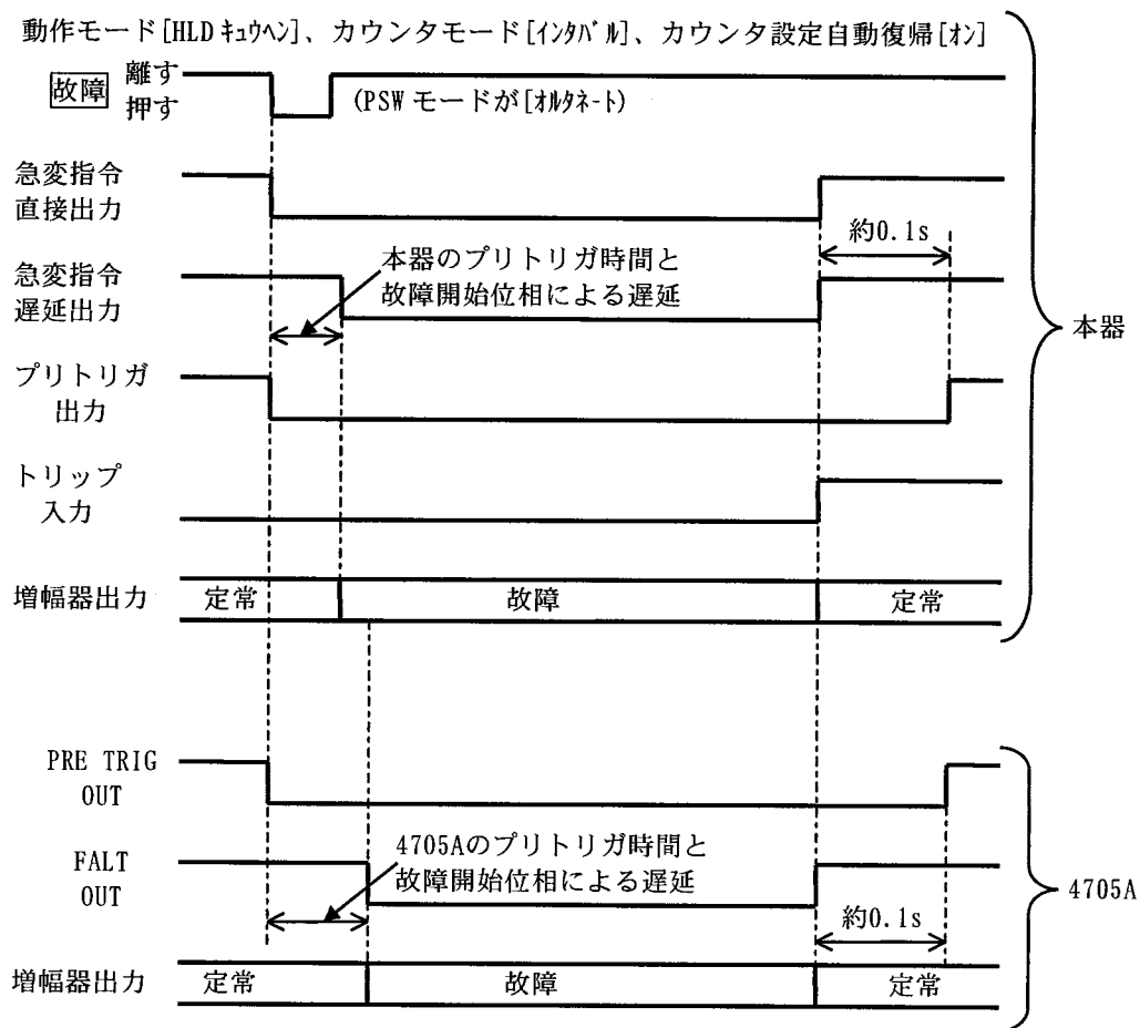
図 4-7 4705A プリトリガ時間、故障開始位相を個別設定の動作
