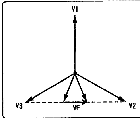
図 3-8 2LS 設定
