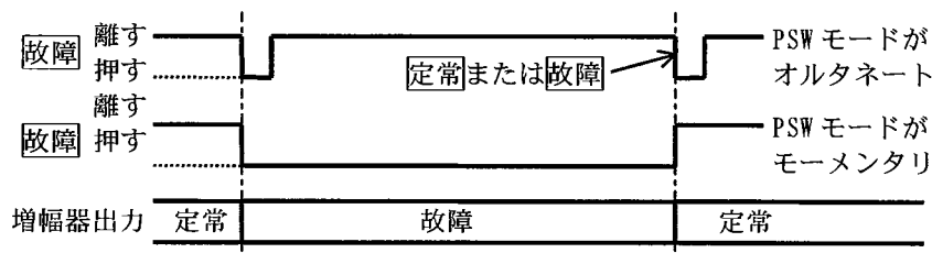
図 3-9 PSWモードの動作
