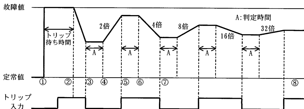
図 3-21 DSK サーチスイープの動作
