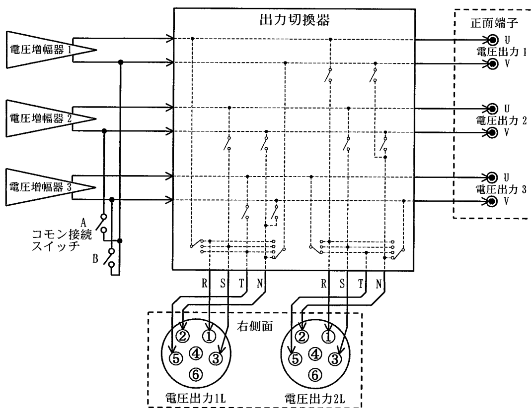
図 3-2 出力切換器の構成
