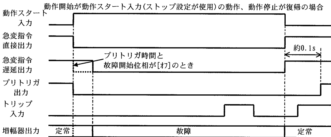
図 3-12 ホールド急変の動作、自動復帰[お]
