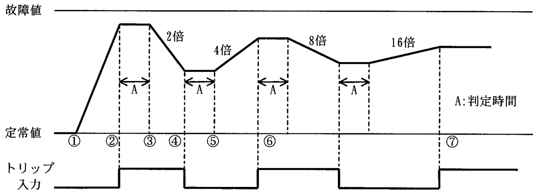
図 3-20 サーチスイープの動作
