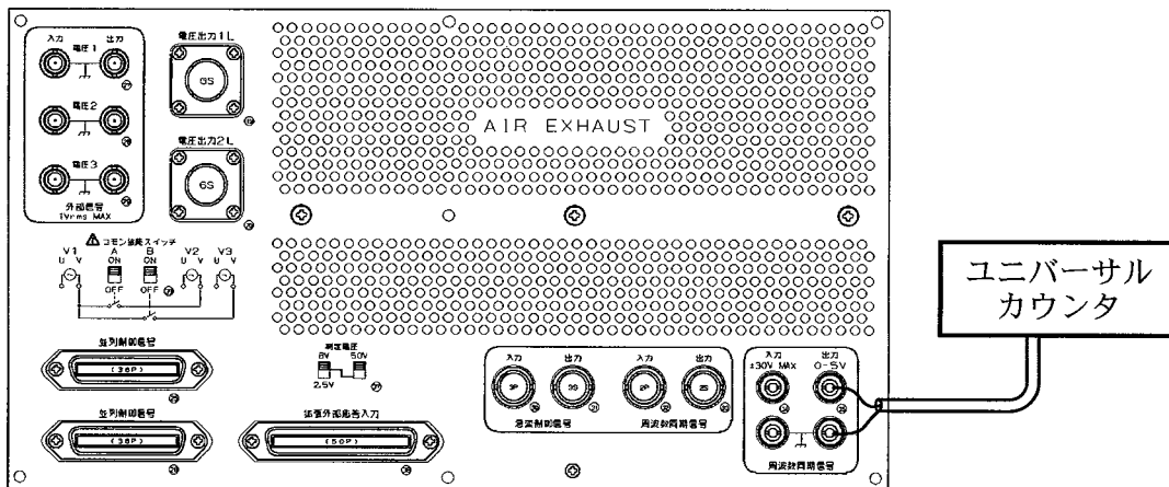
図 8-3 ユニバーサルカウンタの接続(周波数精度)
