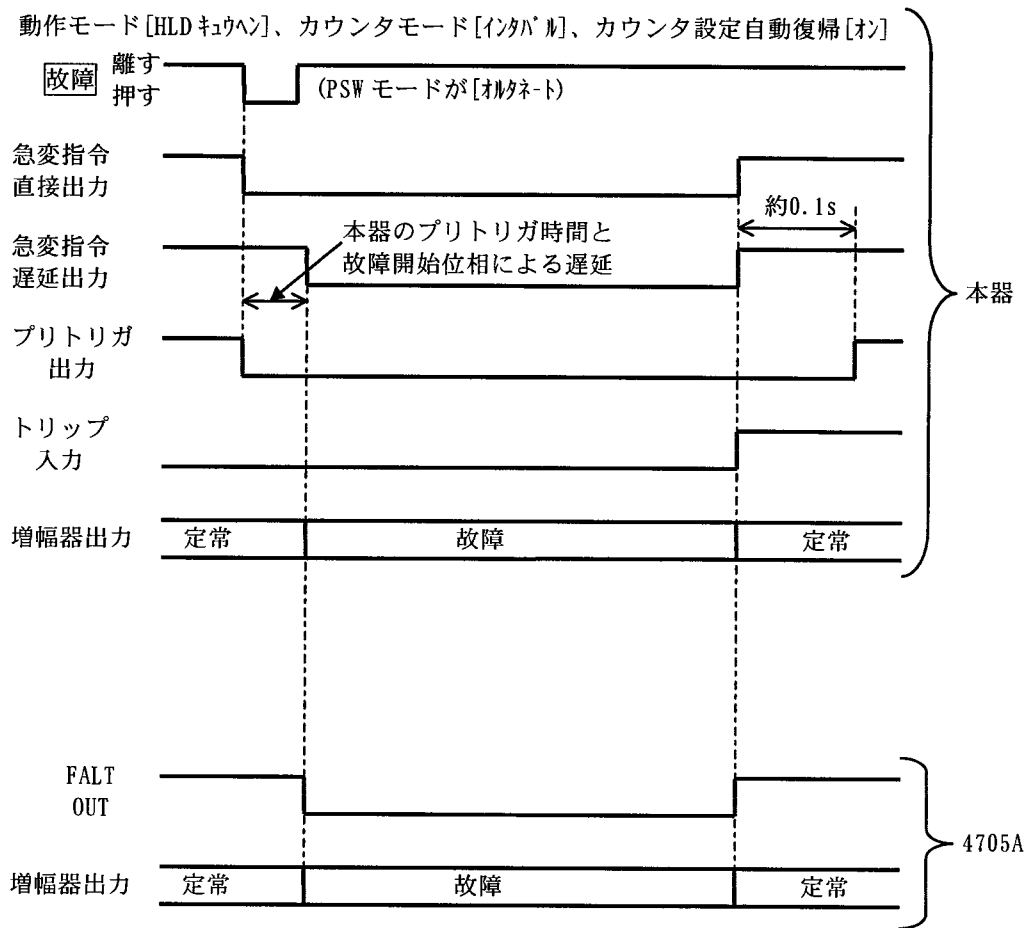
図 4-9 4705A 同時故障急変の動作
