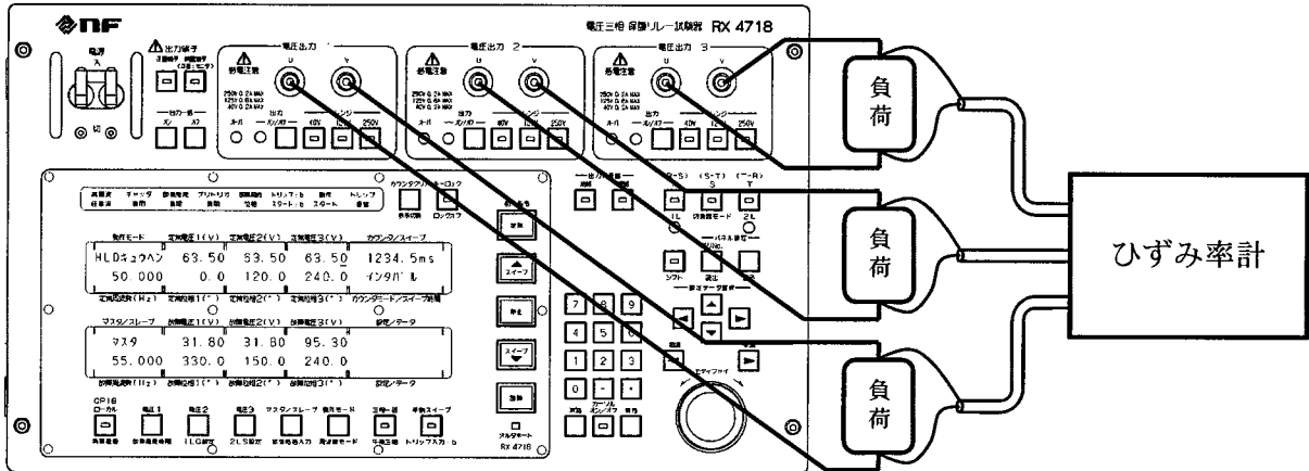
図 8-2 ひずみ率計と負荷の接続
