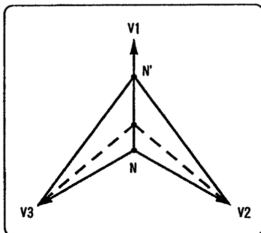
図 3-7 1LG 設定
