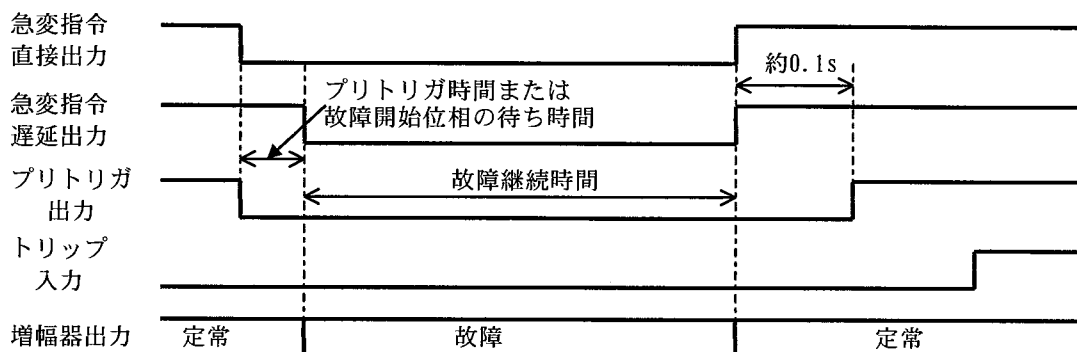
図 3-17 故障継続時間の動作
