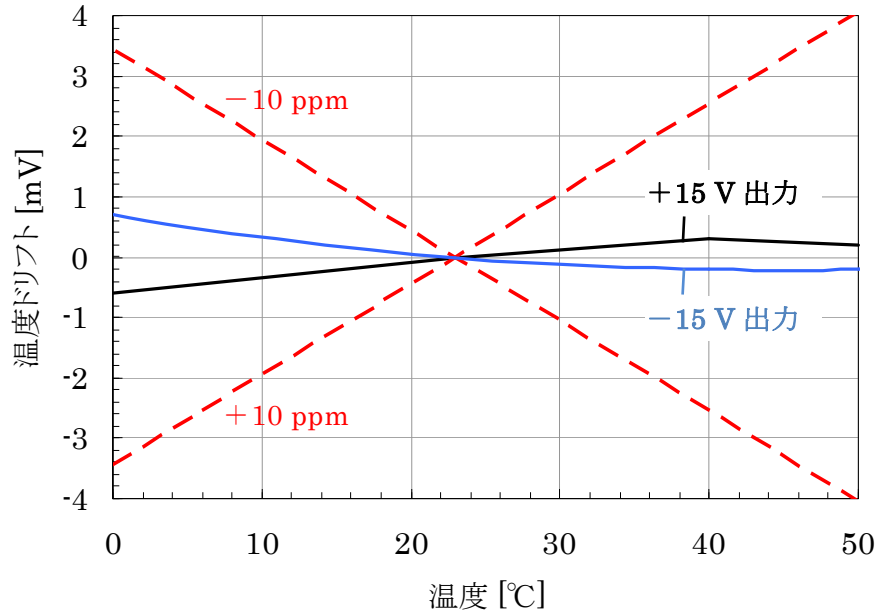
図 6-5 温度ドリフト特性 (定格負荷)
