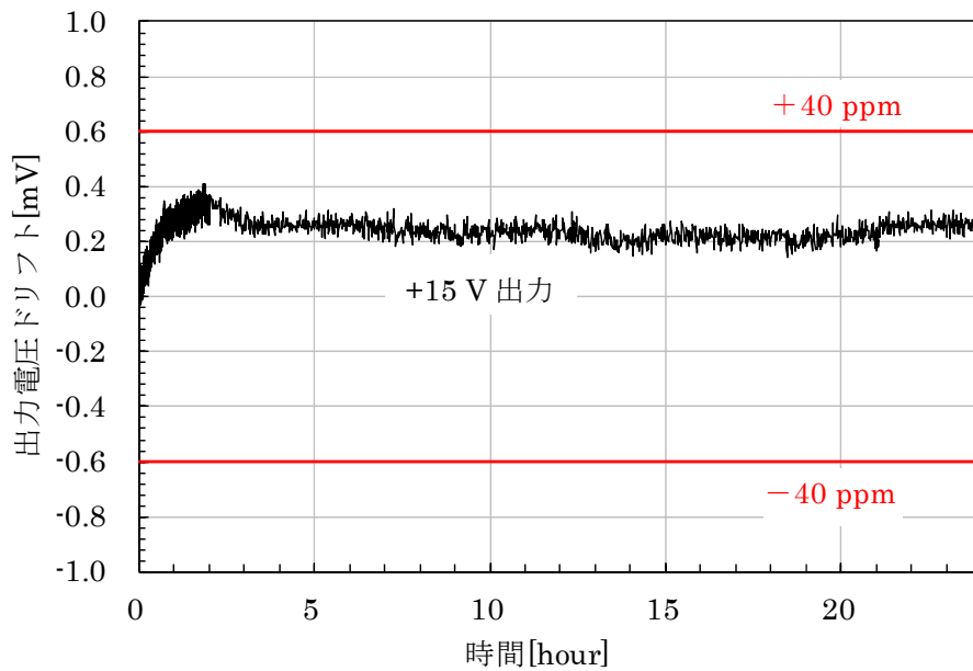
図 6-4 長時間ドリフト (定格負荷, 電源 ON から 30 分後の出力電圧基準)
