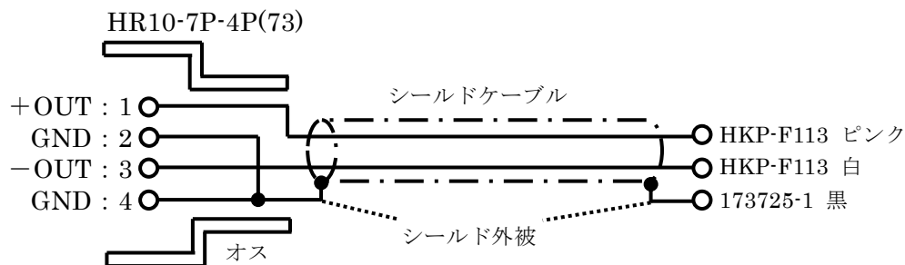
(b) 出力ケーブル B (SA-230F5 を除く全ての SA-200, 400 シリーズ用)
