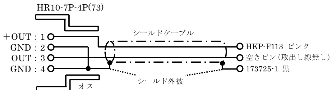
(c) 出力ケーブル C (SA-230F5 用)
