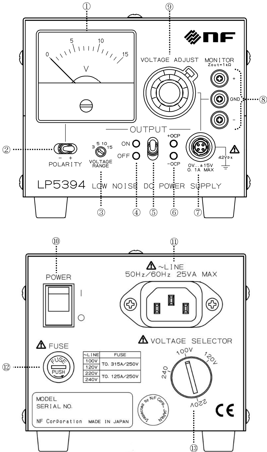
図 3-1 LP5394 の正面・背面パネル図
