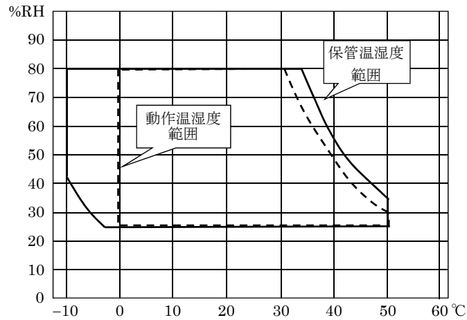
図 5-2 温湿度範囲説明図
