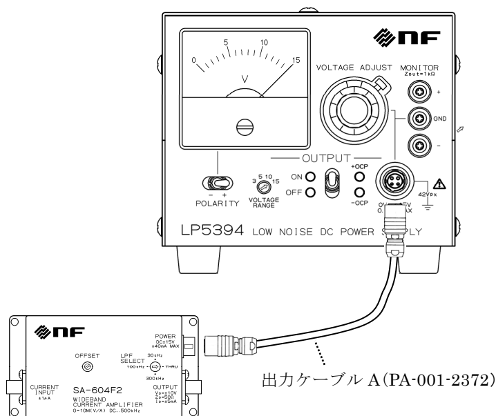
図 3-6 SA-600 シリーズとの接続
