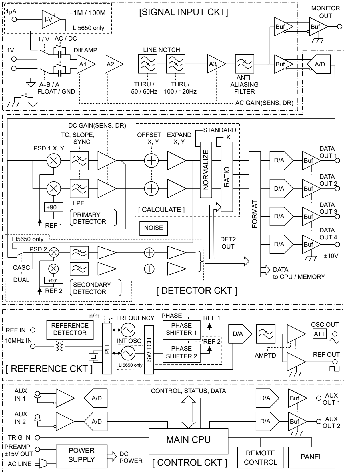
図 1-2 LI5645 / LI5650 ブロック図
