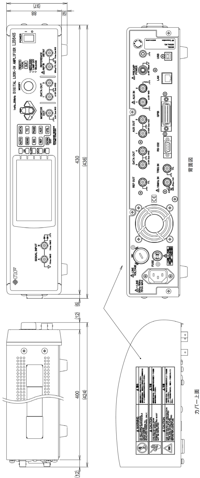
図 9-1 LI 5645 外形寸法図
