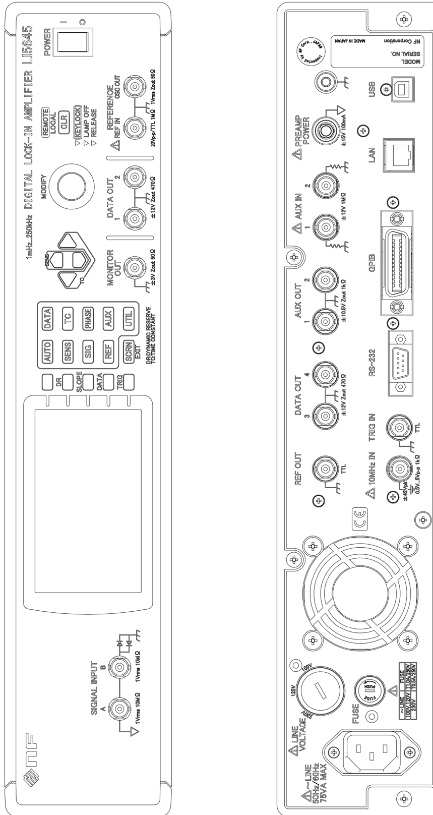
図 9-3 LI 5645 パネル図
