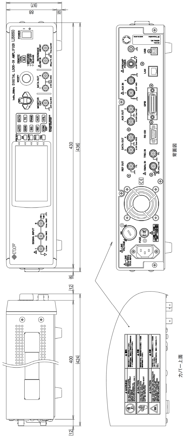
図 9-2 LI 5650 外形寸法図
