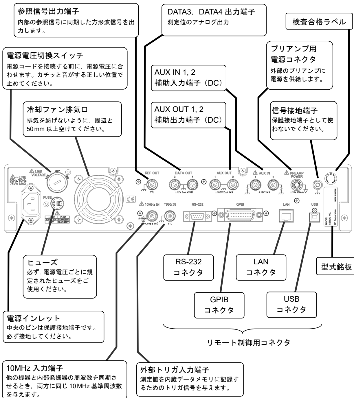
図 3-2 背面パネル
