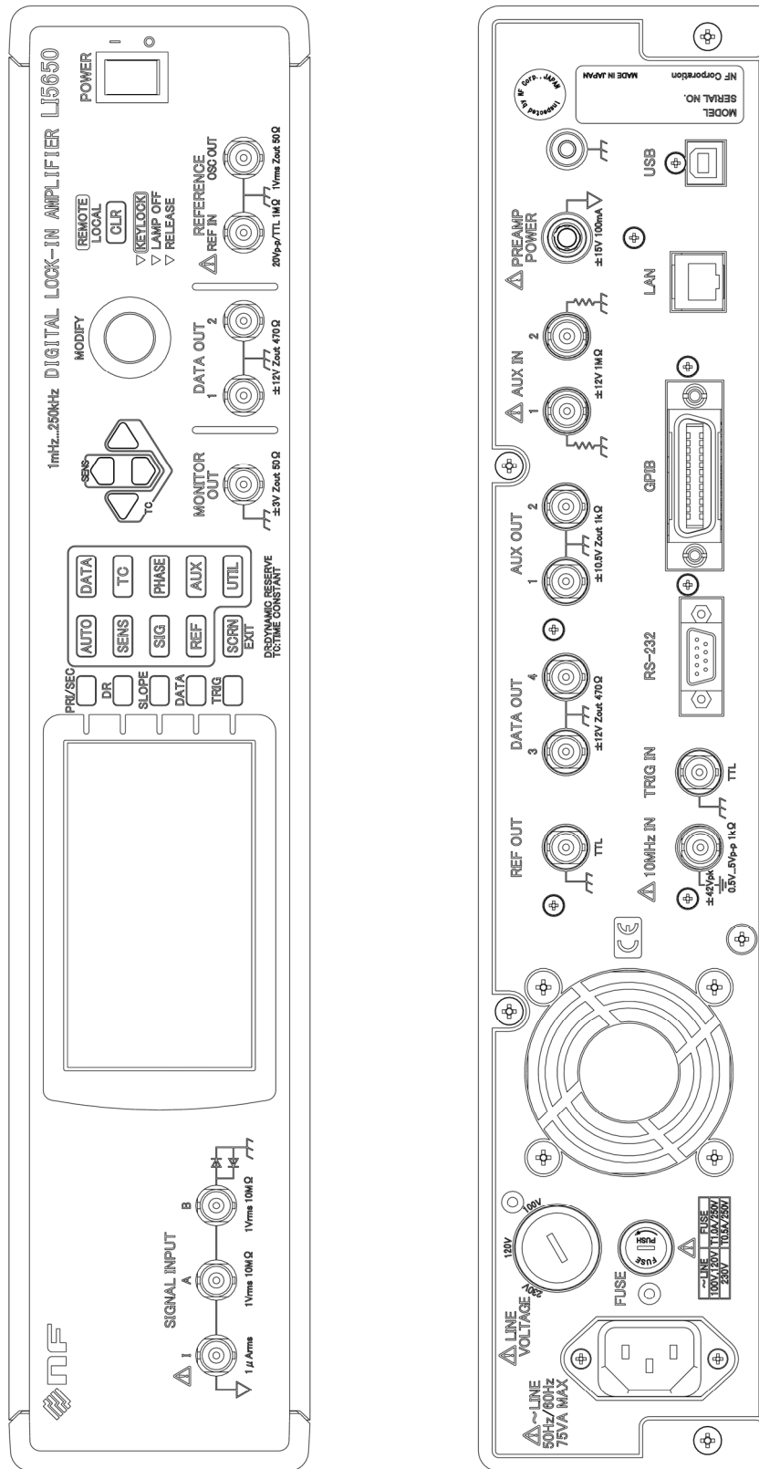
図 9-4 LI 5650 パネル図
