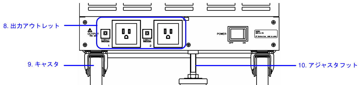
図3-2 各部の名称（フロント）出力アウトレットオプションあり（キャスタタイプ）
