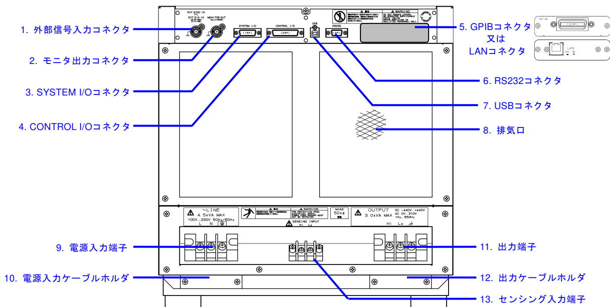
図3-3 各部の名称 (リア) (フットタイプ)
