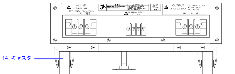
図3-4 各部の名称 (リア) (キャスタタイプ)
