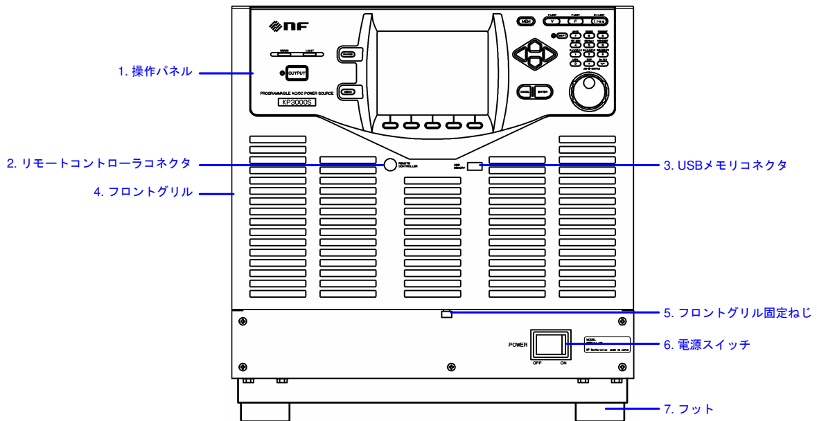
図3-1 各部の名称（フロント）（フットタイプ）
