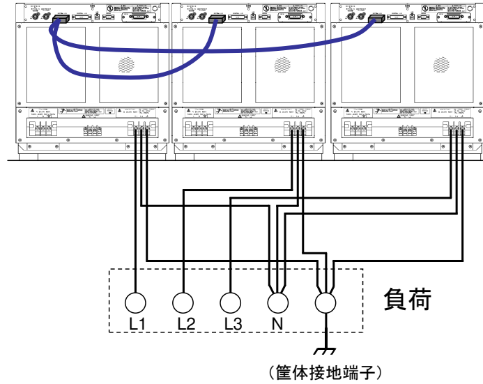
(a) 三相4線接続
