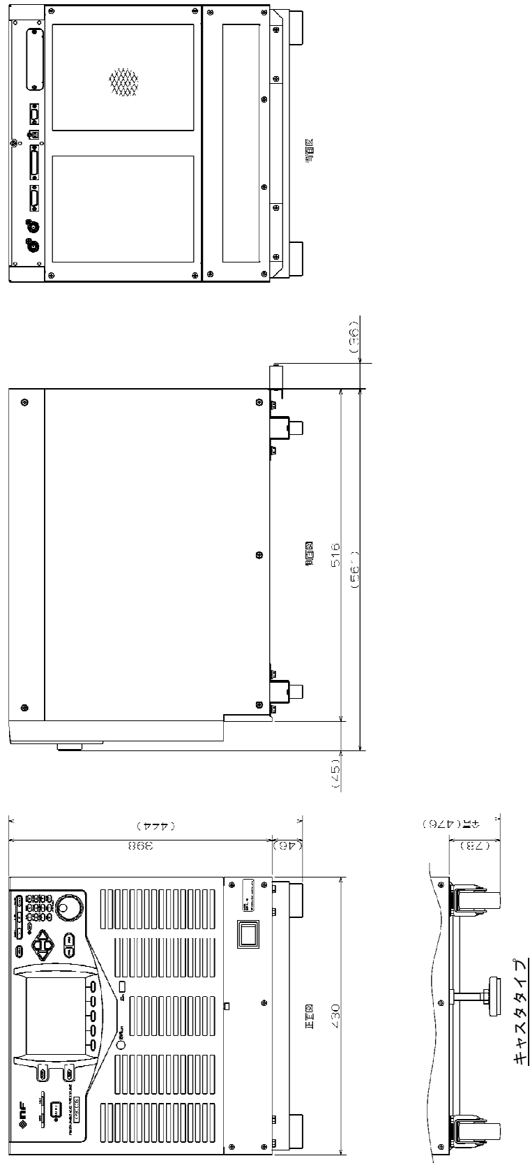
図10-2 外形寸法
