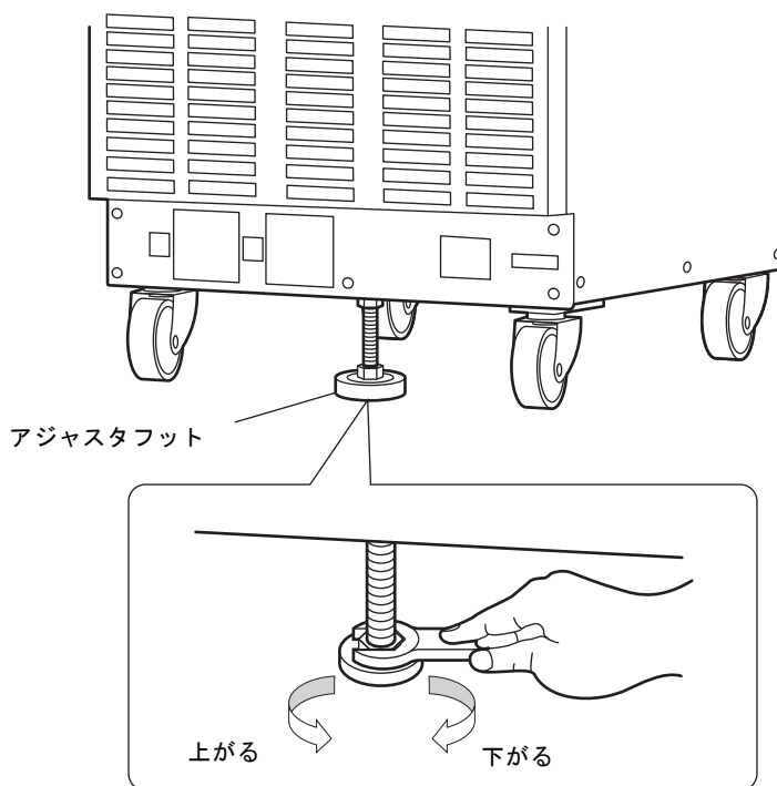
図2-1 アジャスタフット（キャストタイプを含む）の使用方法
