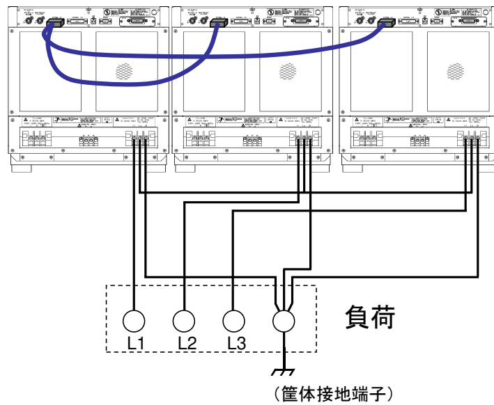
(b) 三相3線接続
