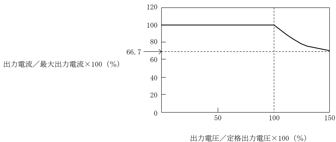
図 5-1 出力電圧 対 出力電流特性
