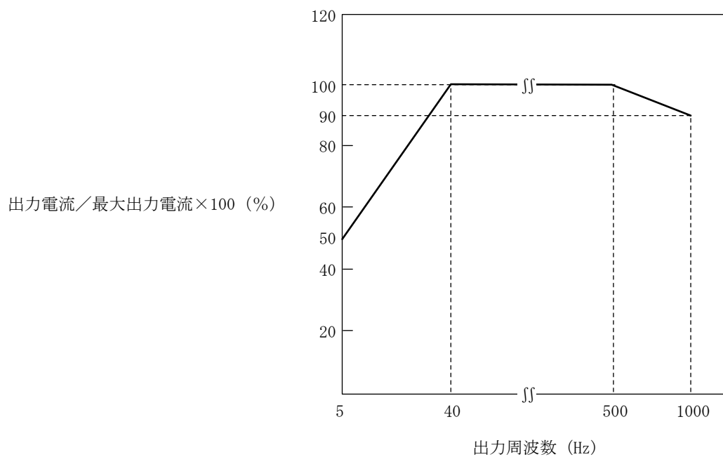
図 5-2 出力周波数 対 出力電流特性
