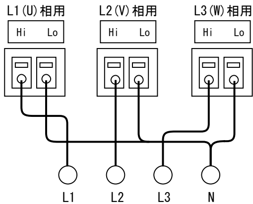
三相/单相 3 線モード時
