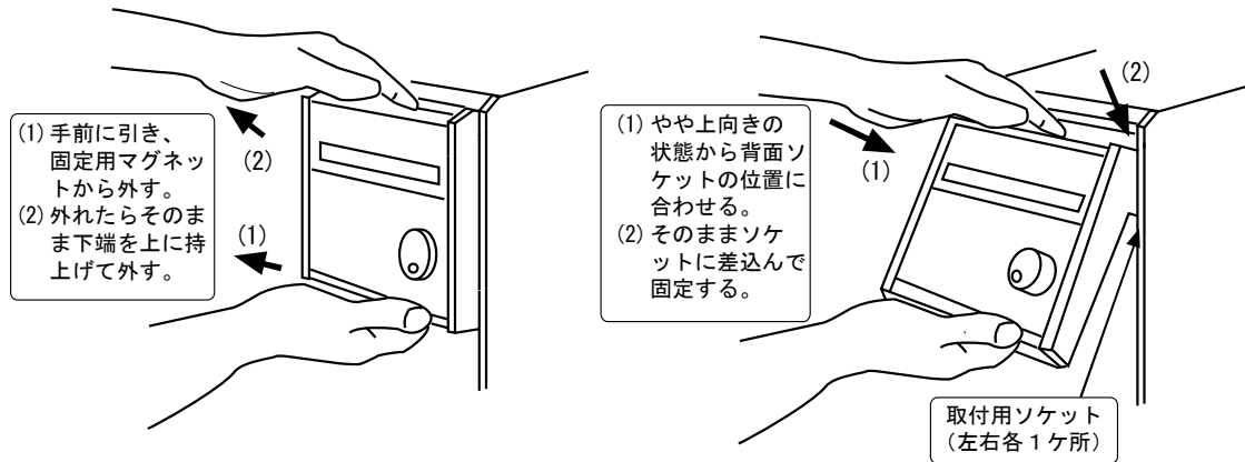
図 4-1 コントロール部の外し方
