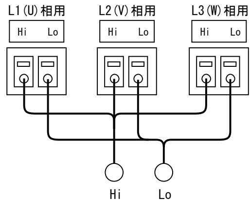
单相 2 線モード時
