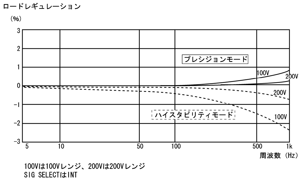
図 5-7 ロードレギュレーション 対 周波数特性
