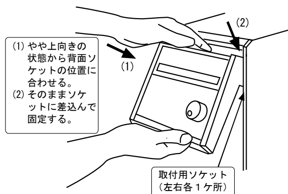
図 4-2 コントロール部の上向き固定方法
