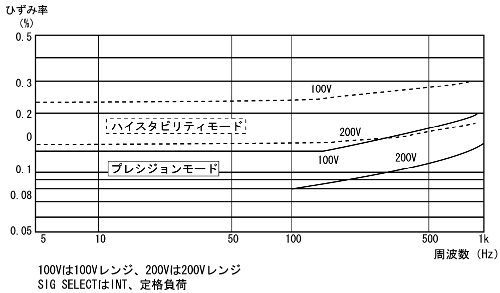
図 5-6 全高調波ひずみ率 対 周波数特性
