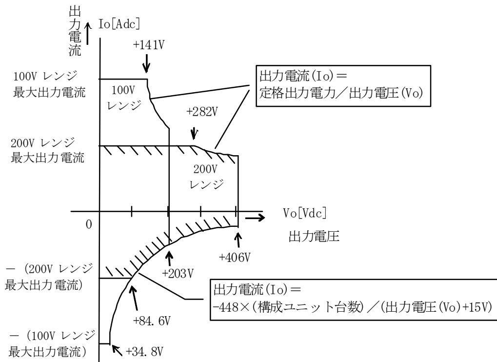
直流出力モード出力電圧対出力電流特性
