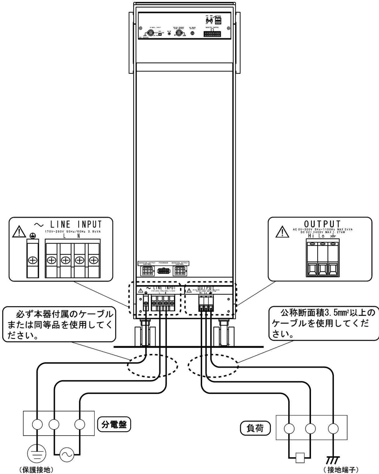
図 3-1 ES020ES の接続方法
