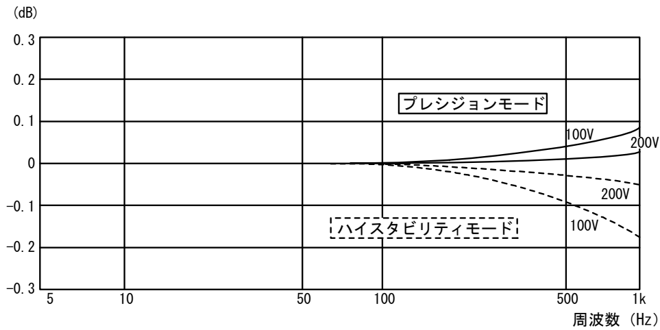
図 5-10 出力電圧 対 周波数特性
