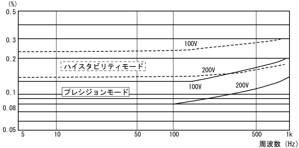
図 5-11 全高調波ひずみ率 対 周波数特性
