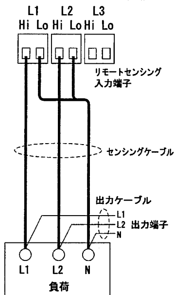
単相三線モード時の接続
