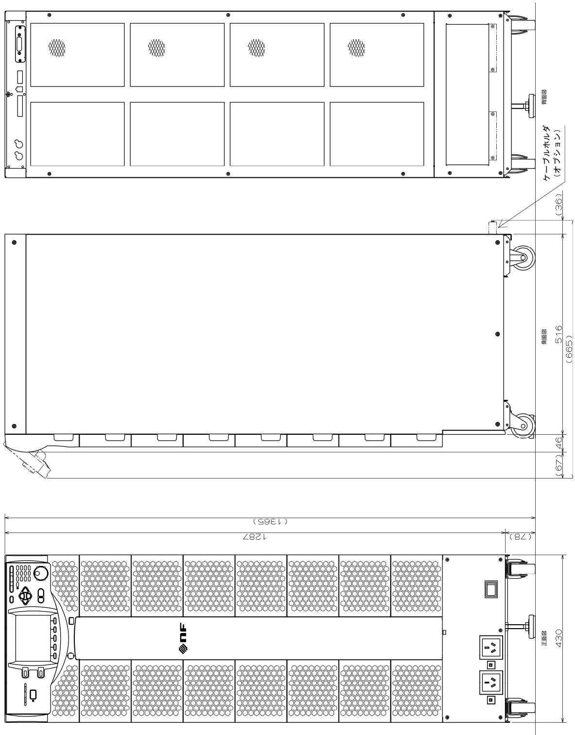
図10-5 DP105KSC, DP120KSC (Type4 キャビネット)
