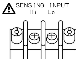
図4-24 センシング入力端子
