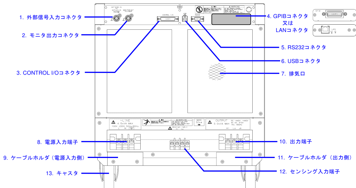
図3-2 各部の名称 (リア)
