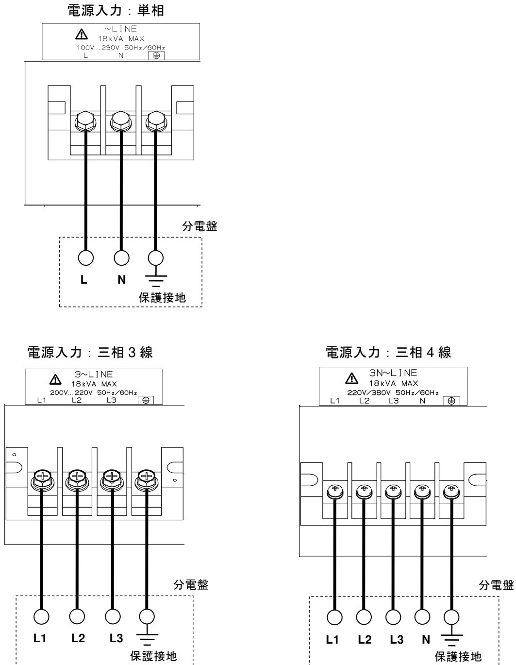
図2-3 電源入力端子
