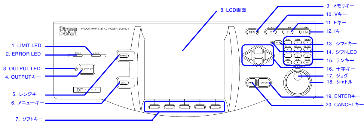
図3-3 各部の名称（操作パネル）
