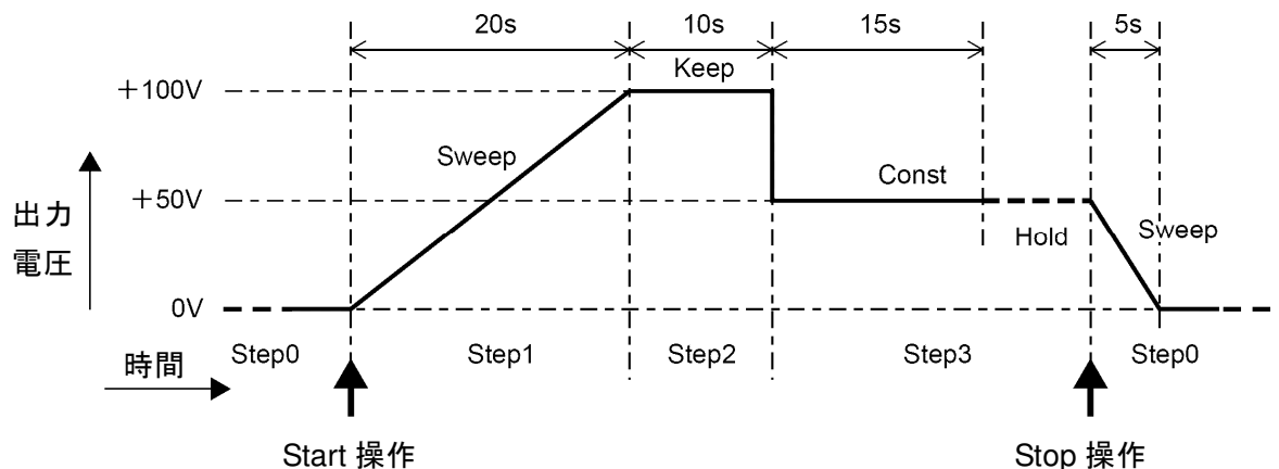
図4-4 シーケンスの例
