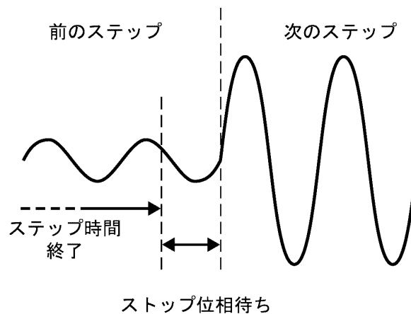
図4-3 ステップ終了位相
