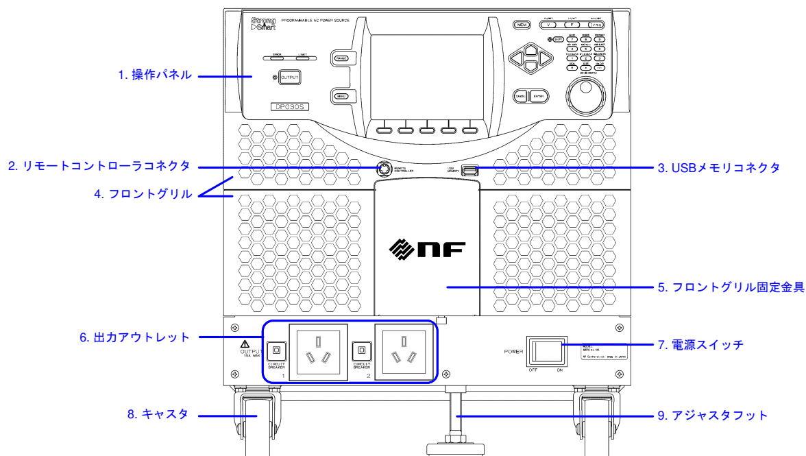
図3-1 各部の名称（フロント）
