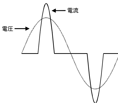
図4-20 高調波成分を多く含む電流波形
