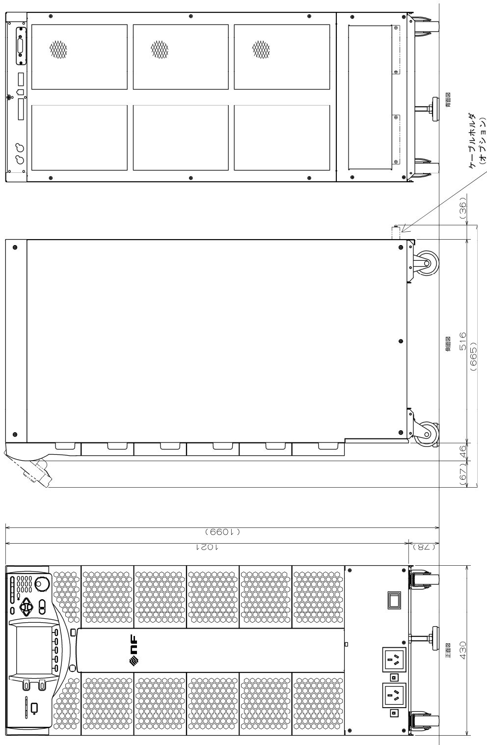
図10-4 DP075KSC, DP090KSC (Type3 キャビネット)
