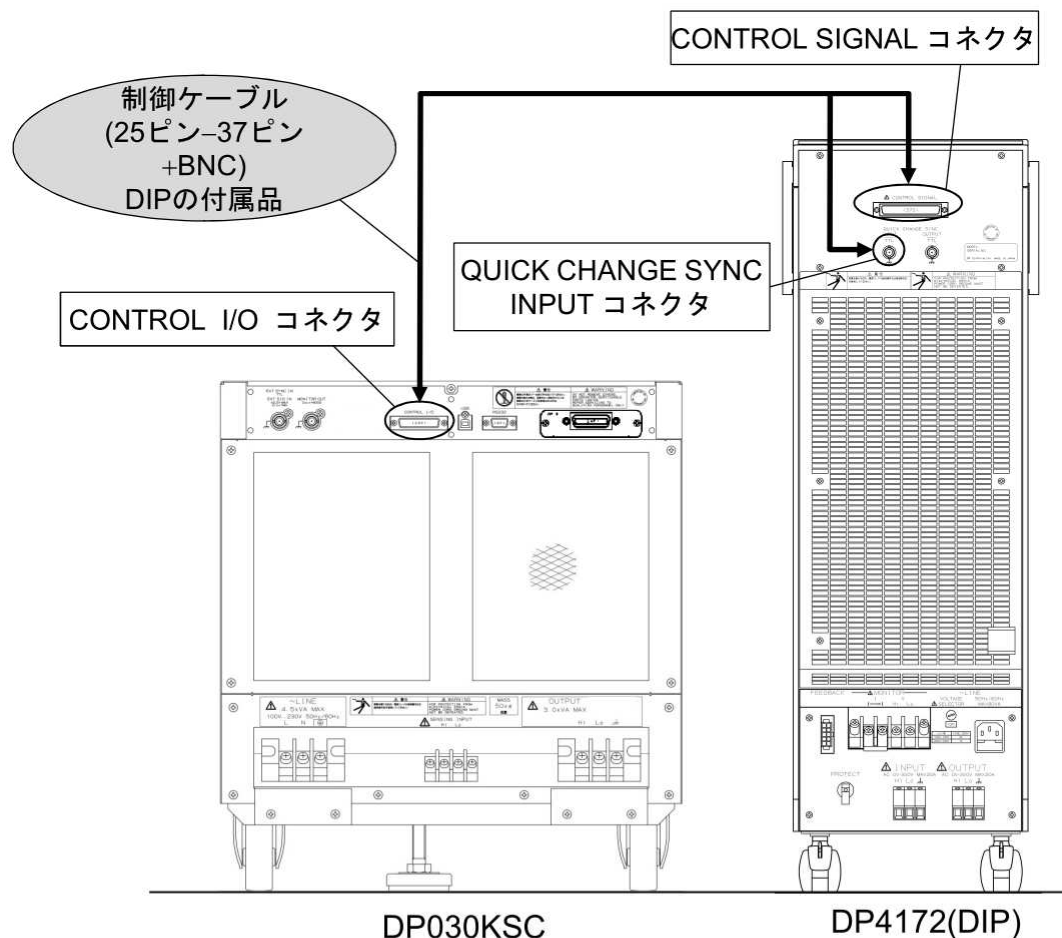
図4-25 DP030KSC と DP4172(DIP)の制御ケーブル接続図
