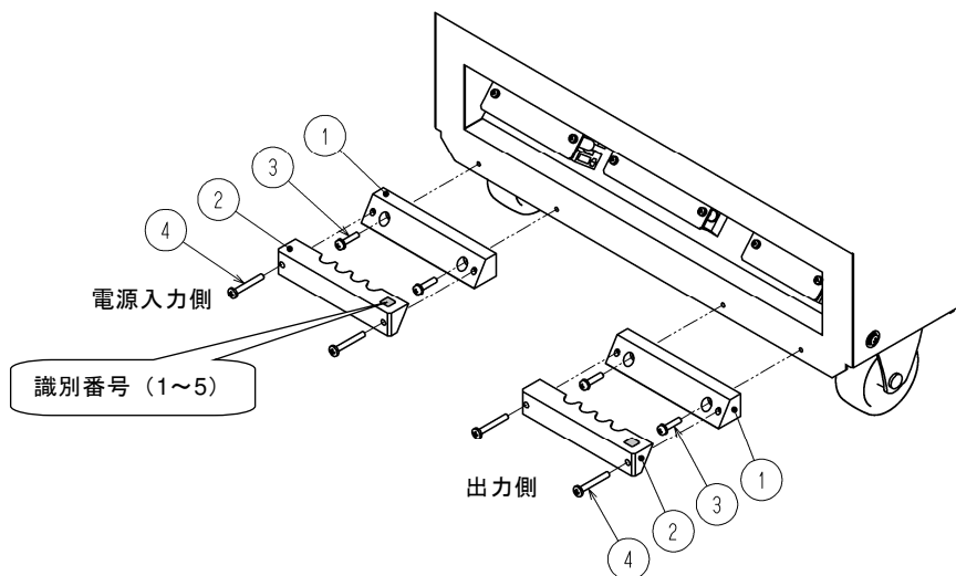
図7-3 ケーブルホルダ取付図
