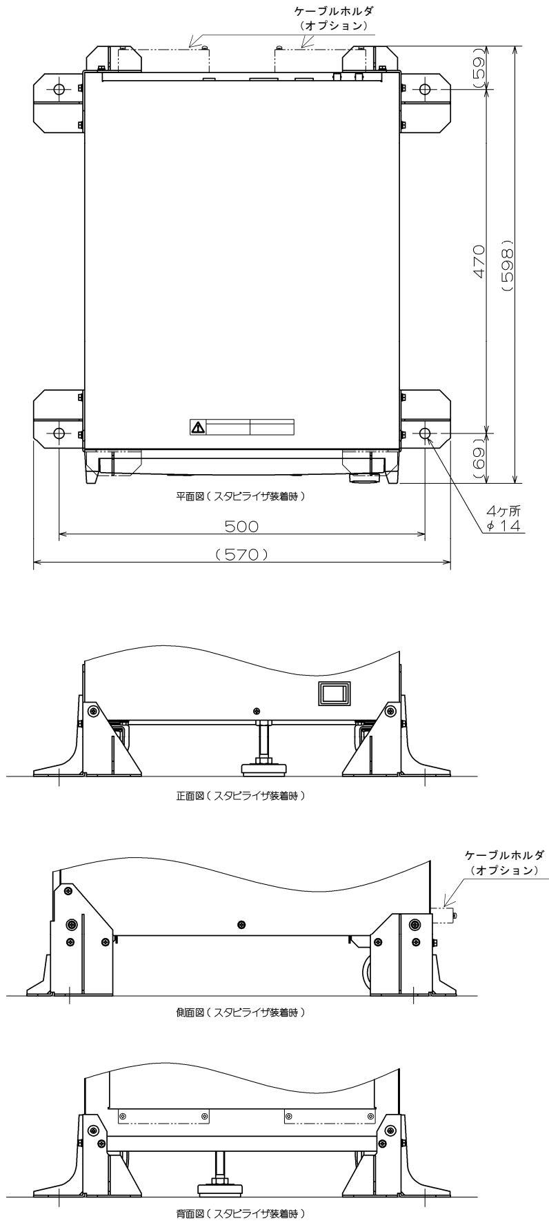
図10-6 スタビライザ装着時 (Type3, Type4 キャビネットのみ)
