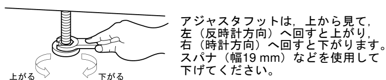
図2-1 アジャスタフットの使用法
