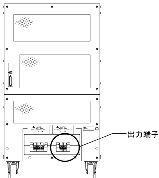
図 2-3 出力端子
