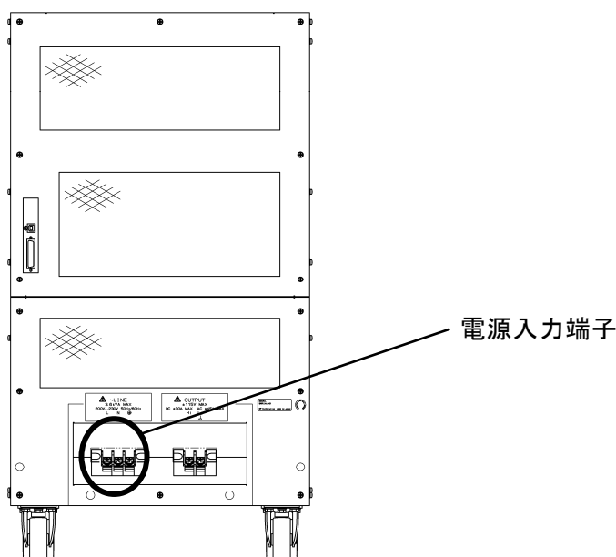
図 2-2 電源入力端子
