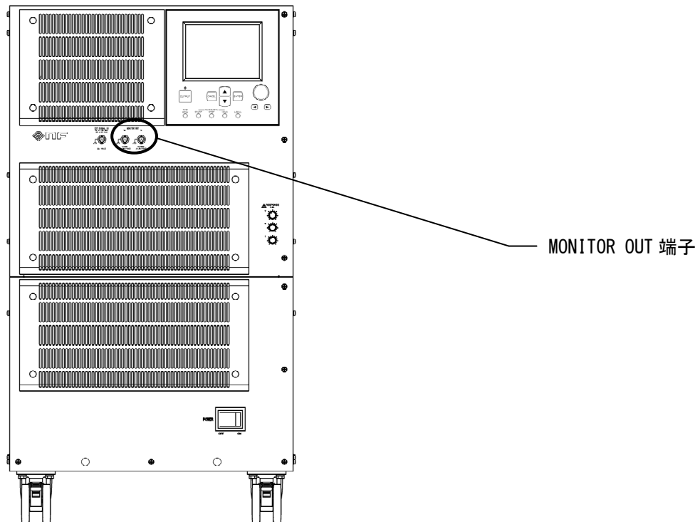
図 4-24 MONITOR OUT 端子
