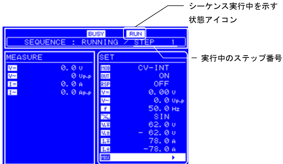
図 4-21 シーケンス実行時の LCD 画面
