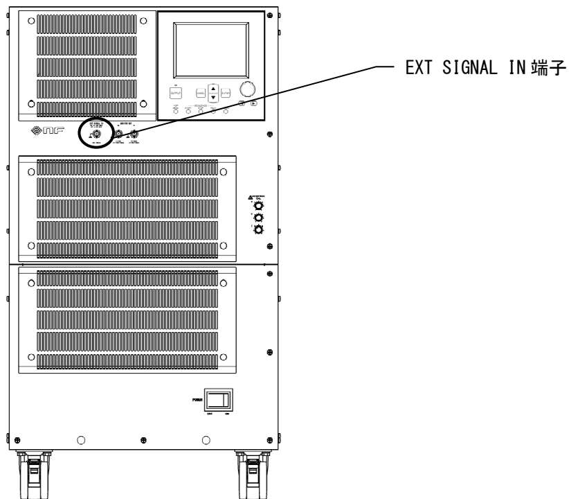
図 2-7 EXT SIGNAL IN 端子
