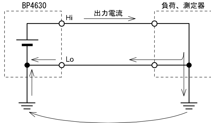
図 2-4 接地された負荷、測定器との接続
