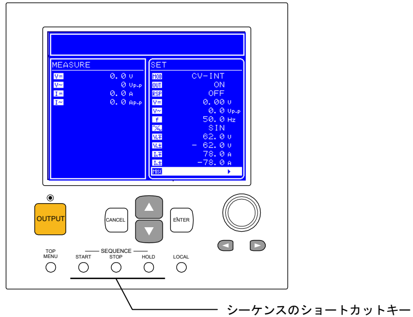
図 4-19 シーケンスのショートカットキー
