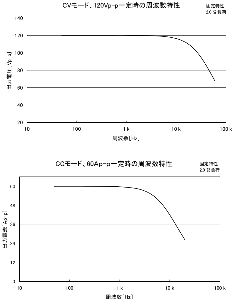
図 4-9 CV, CC モード 2.0 Ω 負荷での周波数特性
