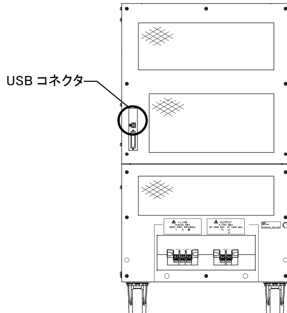
図 2-5 USB コネクタ
