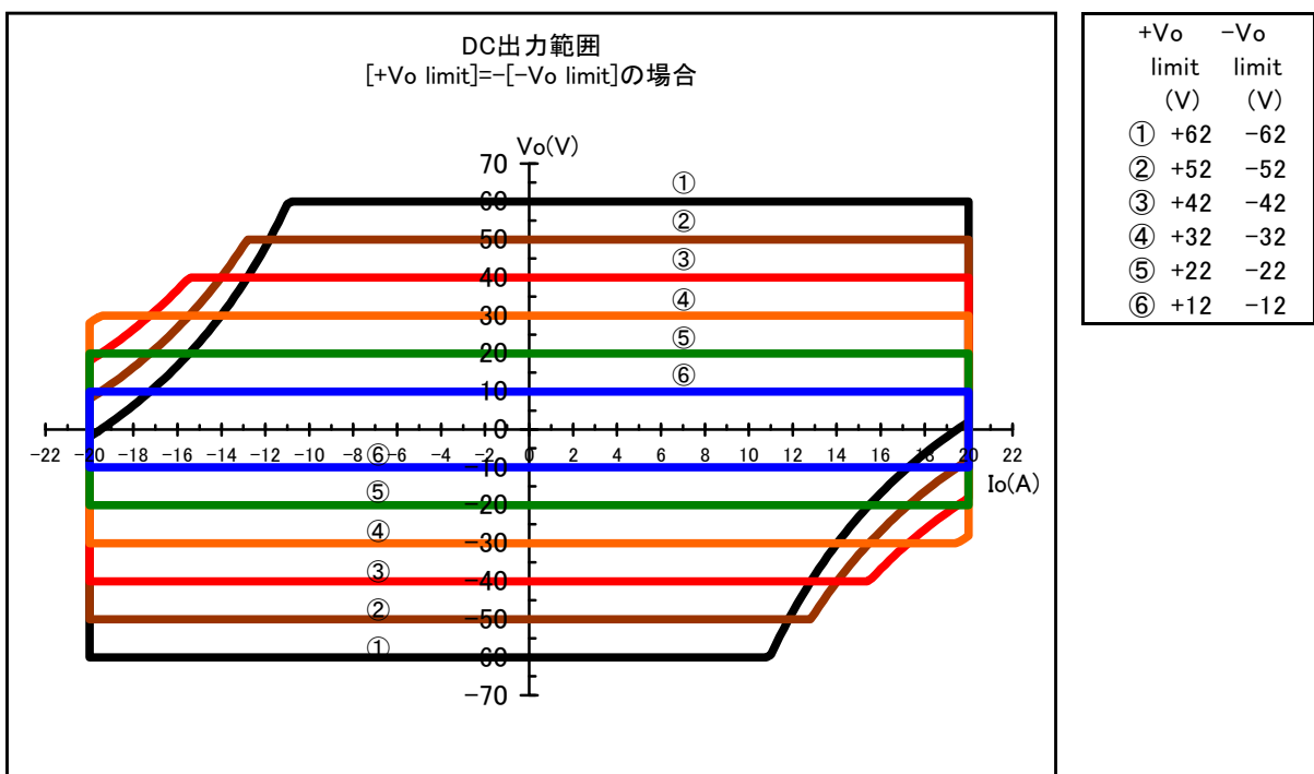
図 8-3 DC 出力範囲（正負電圧リミッタ設定が対称の場合）
