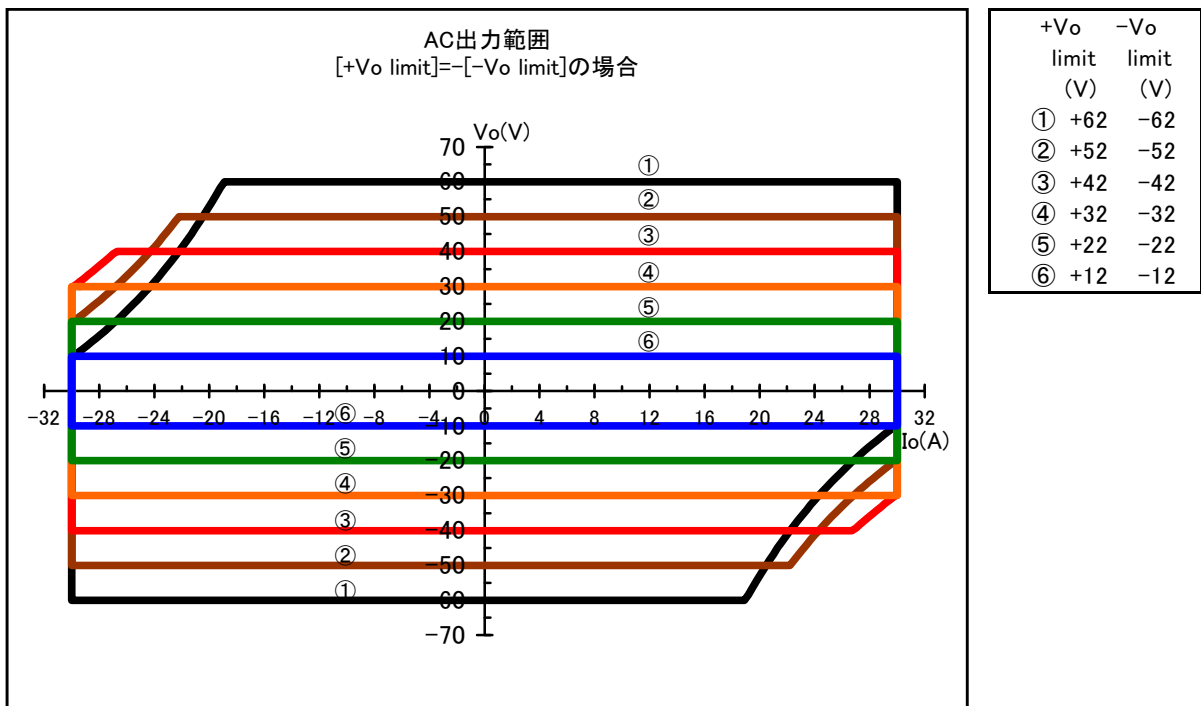
図 8-7 AC 出力範囲 (正負電圧リミッタ設定が対称の場合)
