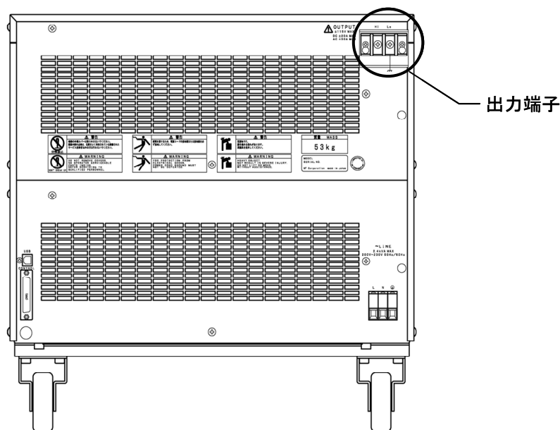
図 2-3 出力端子
