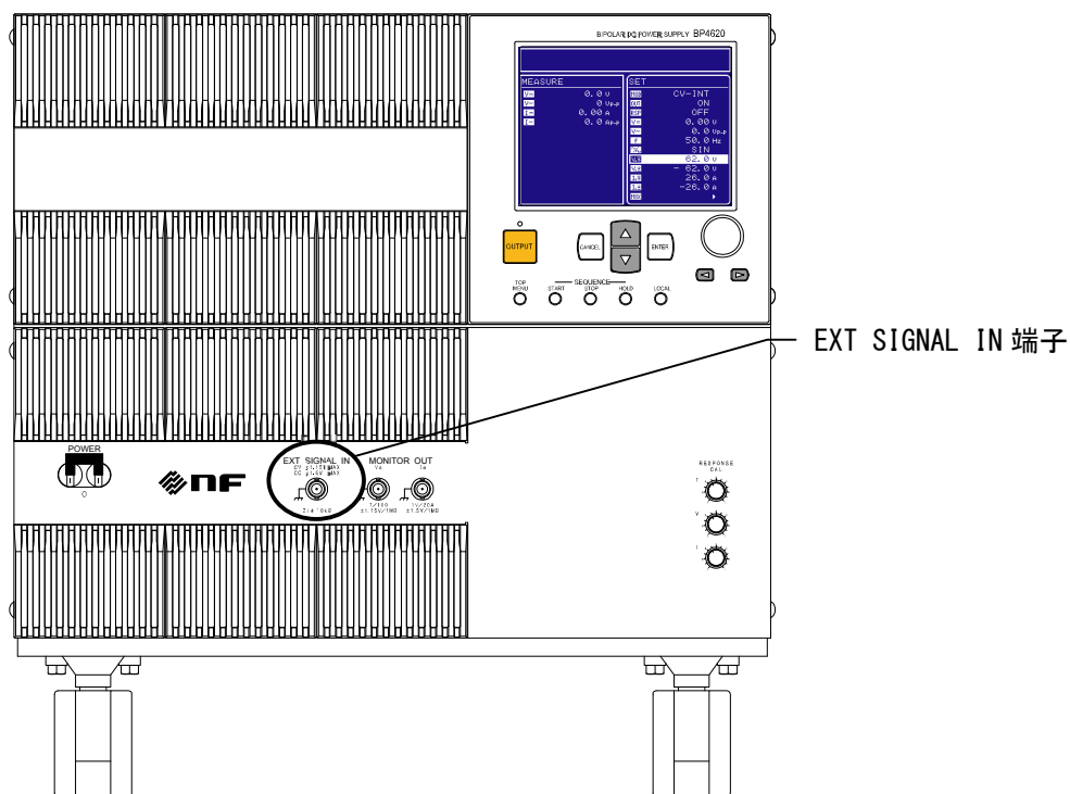
図 4-29 EXT SIGNAL IN 端子
