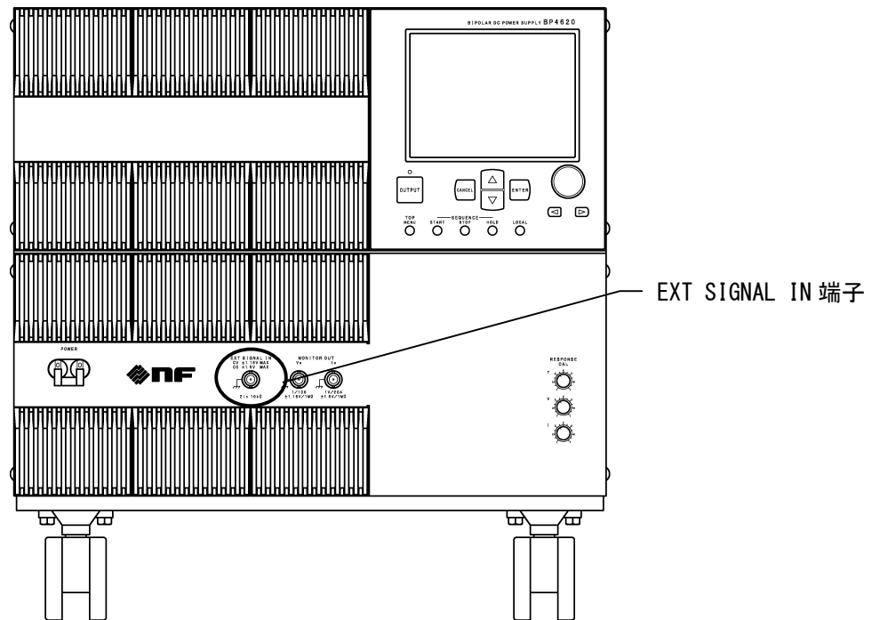
図 2-8 EXT SIGNAL IN 端子
