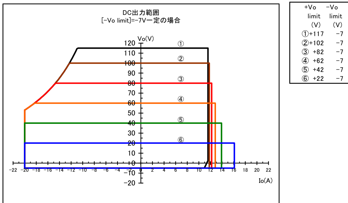
図 4-11 DC 出力範囲（負電圧リミッタ設定が-7 V一定の場合）
