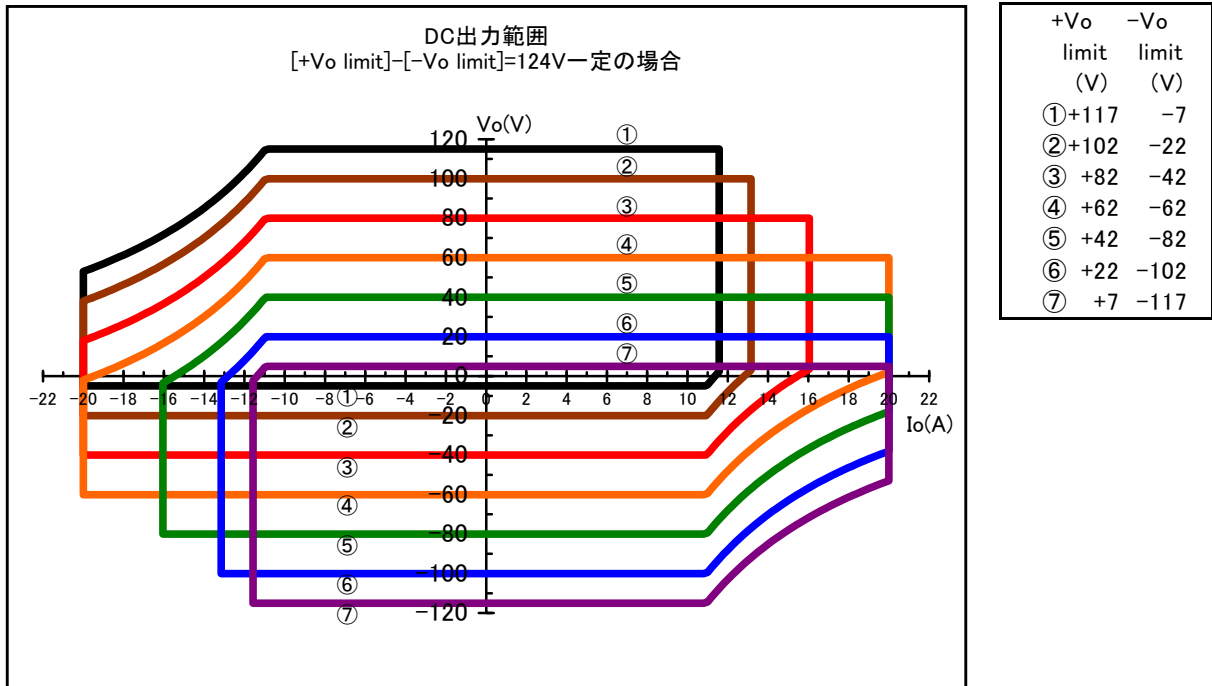
図 8-2 DC 出力範囲（正負電圧リミッタ設定差が 124 V 一定の場合）
