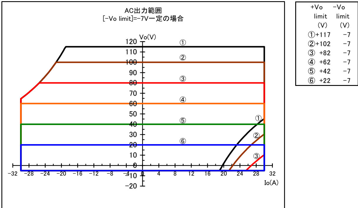
図 8-8 AC 出力範囲 (負電圧リミッタ設定が-7 V 一定の場合)
