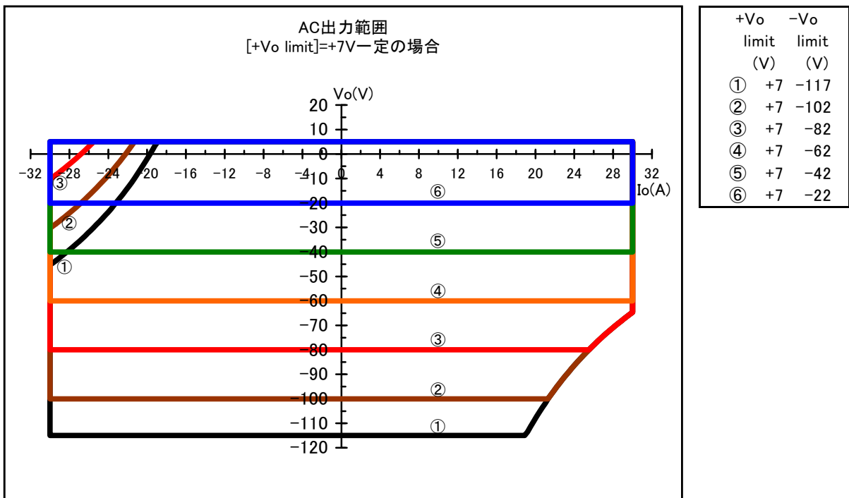
図 8-9 AC 出力範囲 (正電圧リミッタ設定が+7 V 一定の場合)
