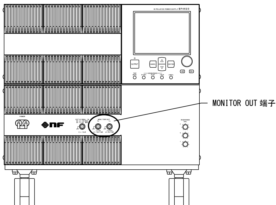
図 2-9 MONITOR OUT 端子
