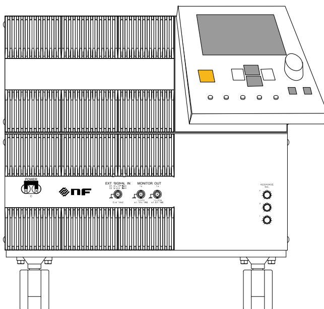
図 3-1 操作パネル部の持ち上げ
