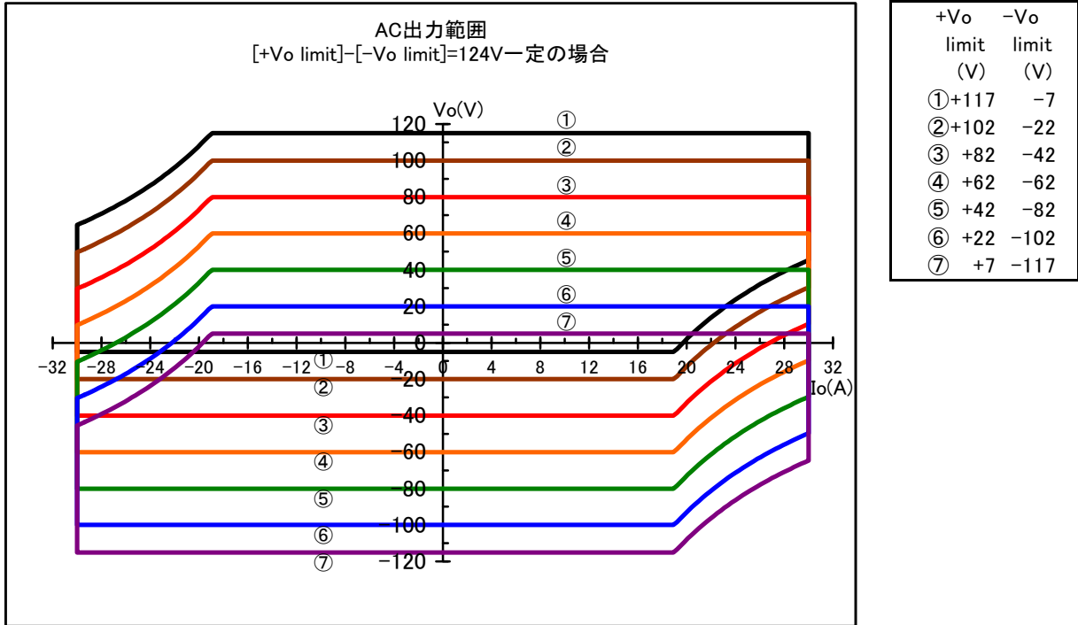
図 8-6 AC 出力範囲 (正負電圧リミッタ設定差が 124 V 一定の場合)
