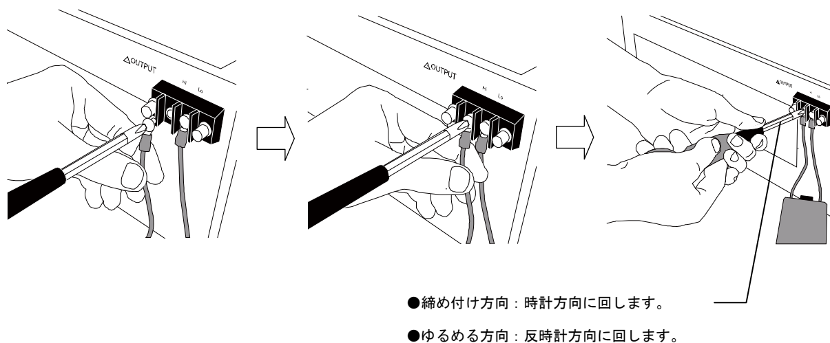
図 2-5 出力端子への接続
