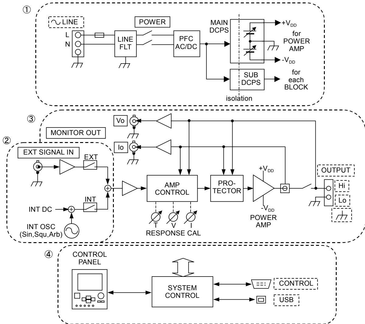
図 1-1 ブロック図
