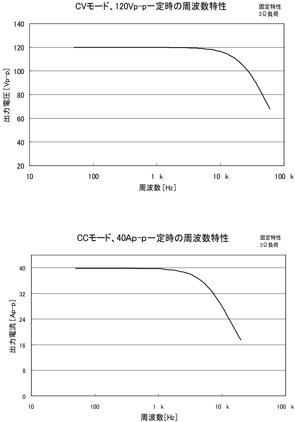
図 4-9 CV, CC モード 3 Ω 負荷での周波数特性
