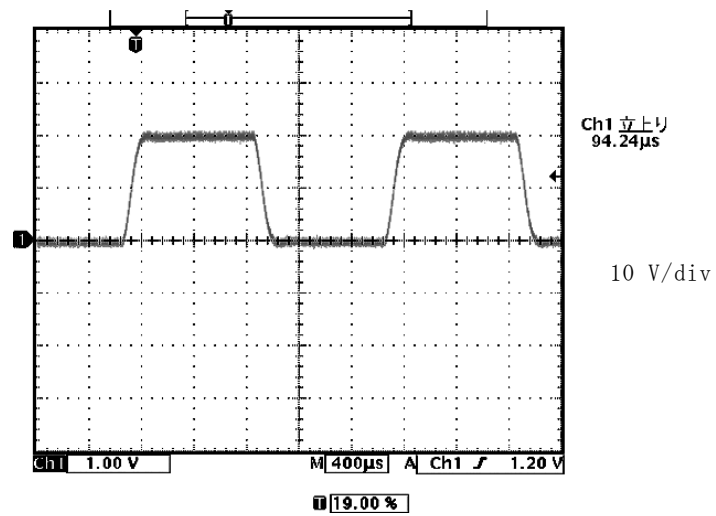
図 4-25 CV モード／容量性負荷時の出力電圧波形 ( C=100 \mu\text{F} )
