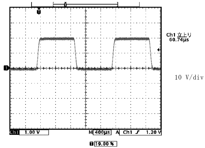
図 4-24 CV モード／容量性負荷時の出力電圧波形 ( C=50 \mu\text{F} )
