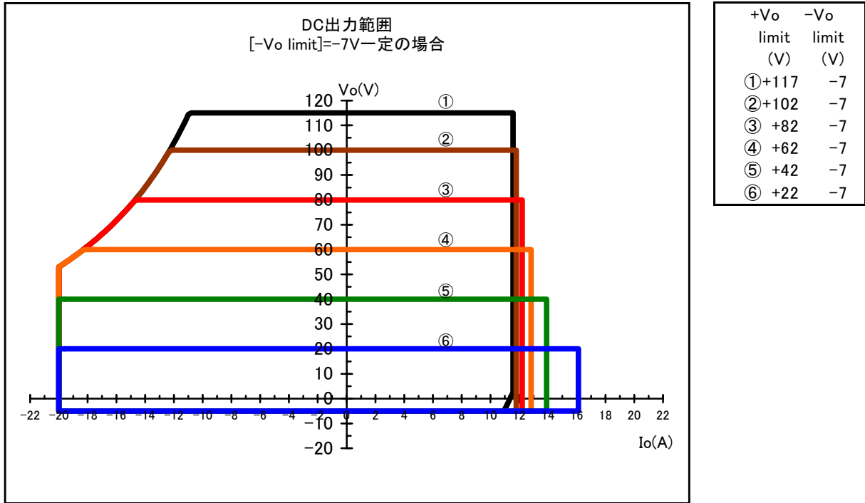
図 8-4 DC 出力範囲 (負電圧リミッタ設定が-7 V 一定の場合)
