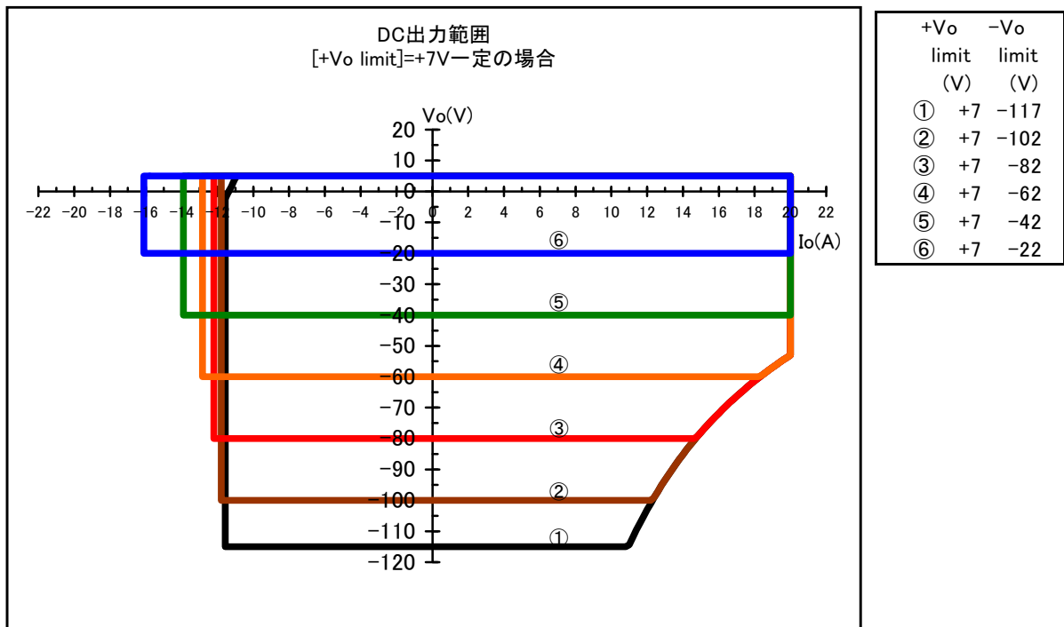
図 8-5 DC 出力範囲 (正電圧リミッタ設定が+7 V 一定の場合)
