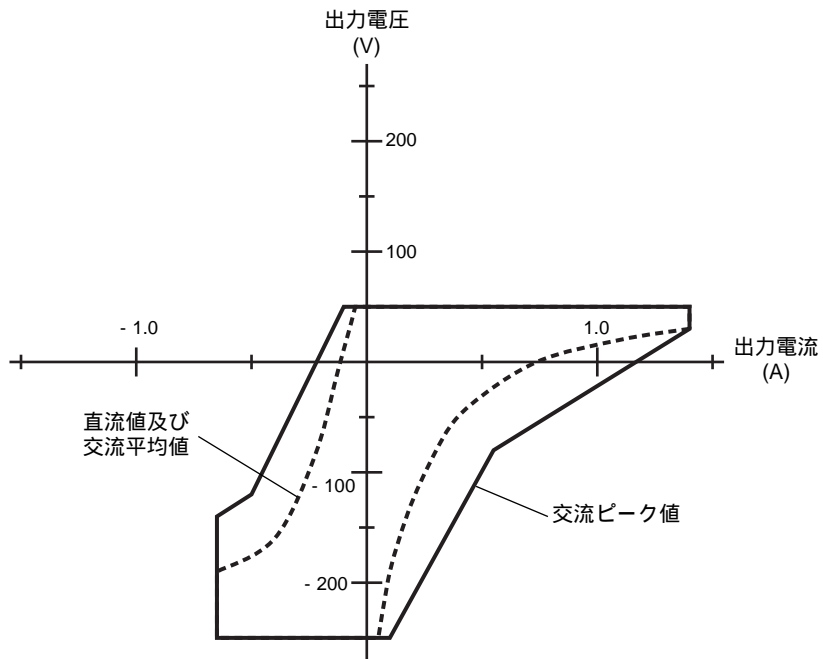
図 4-3 動作領域 (-250 ~ +50 V レンジ)
