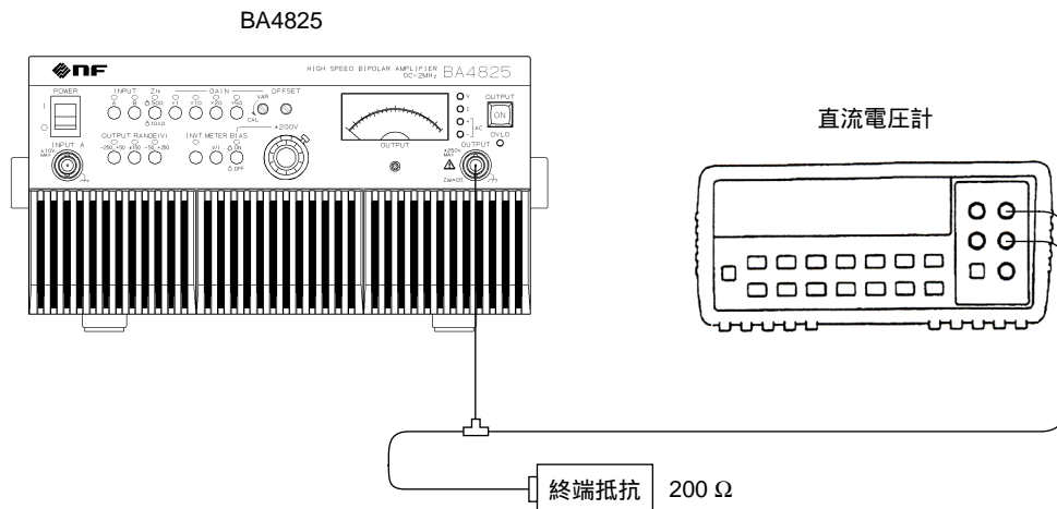
図 6-6 バイアス加算電圧の測定
