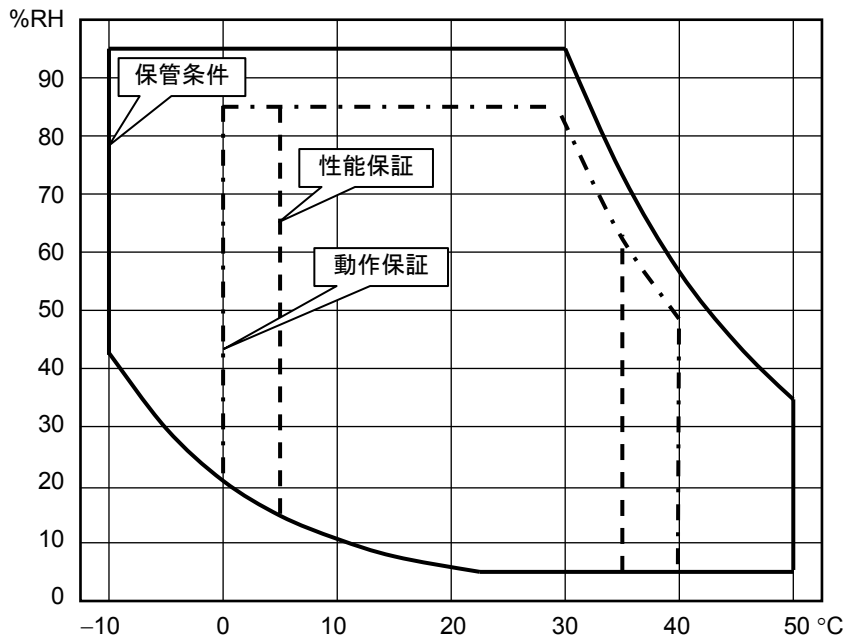
図 7-3 周囲温度, 湿度範囲
