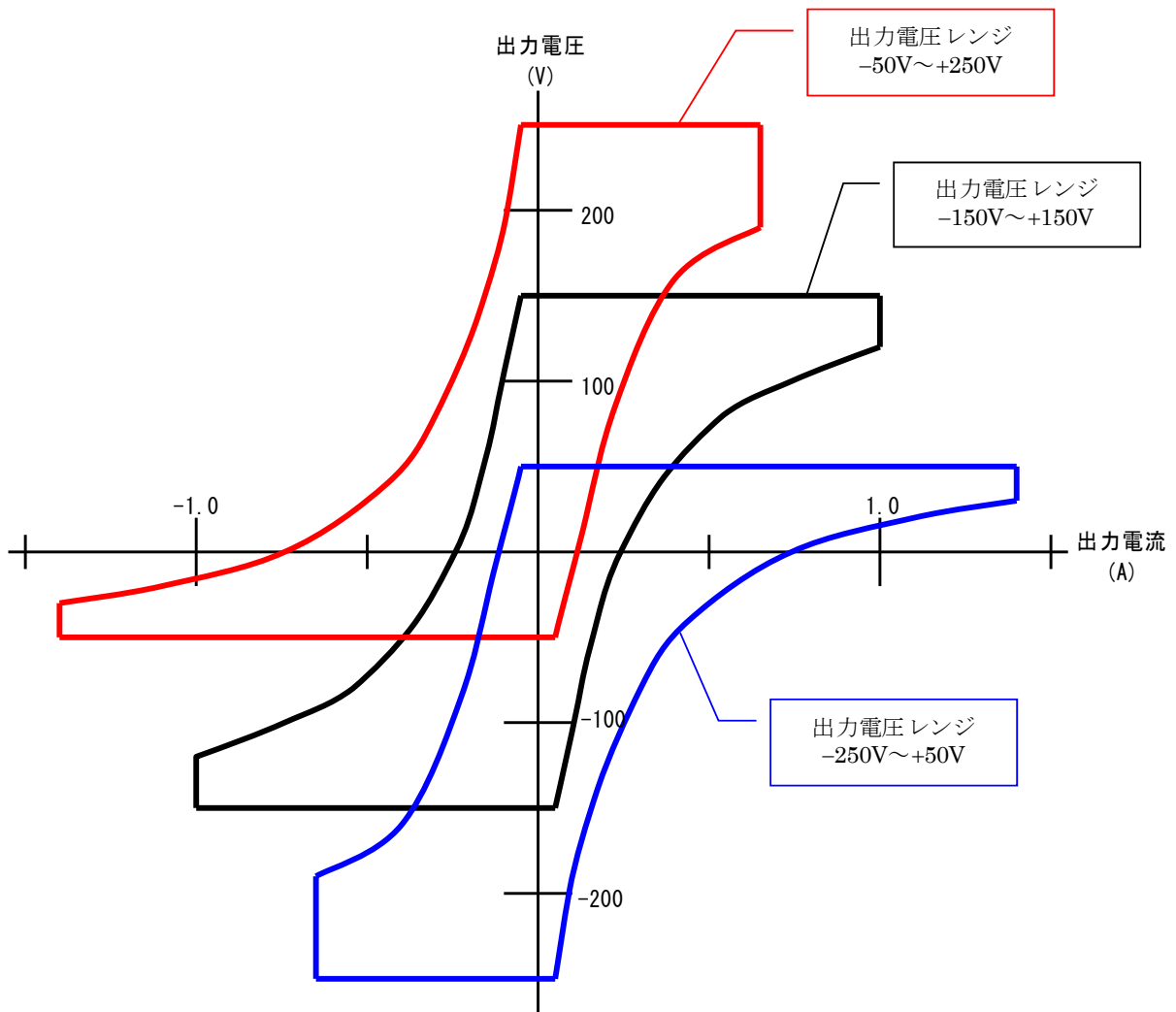
図 7-2 出力電圧・電流範囲 (DC)
