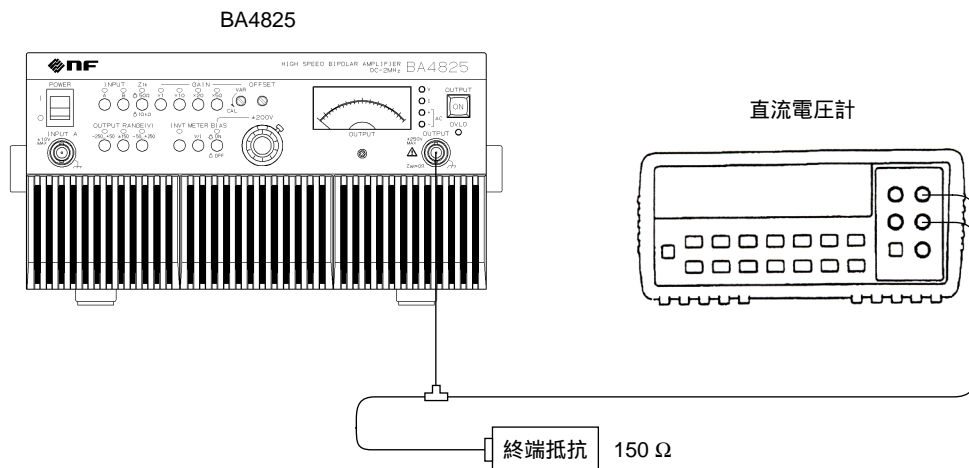
図 6-3 最大出力電力の測定
