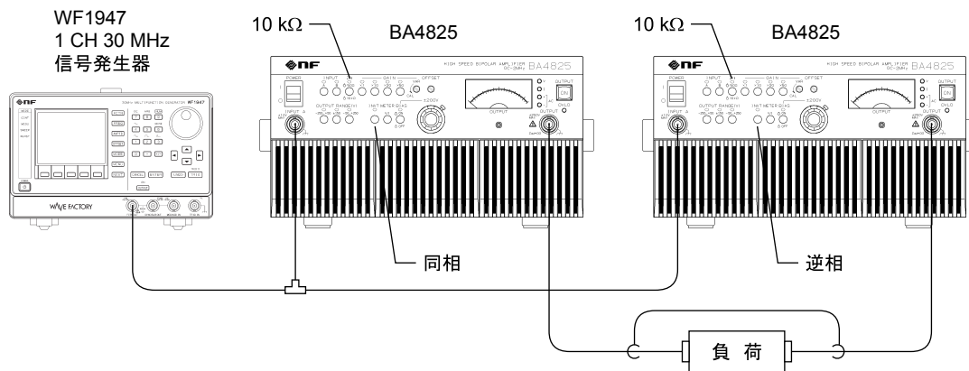
図 4-5 2 台の BA4825 使用時の接続
