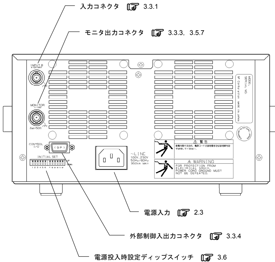
図 3-2 BA4825 リアパネル
