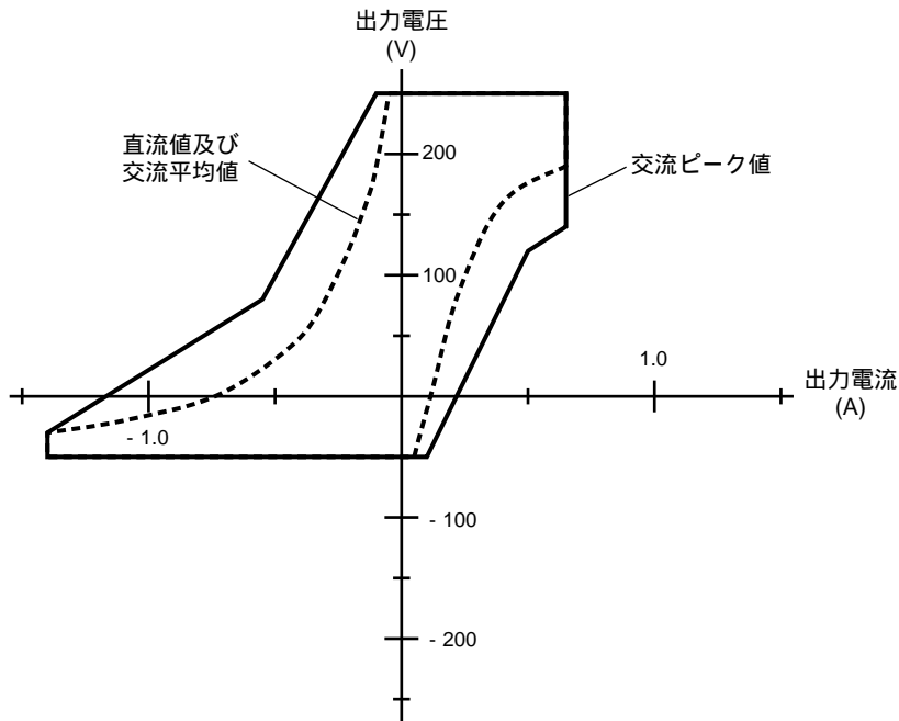
図 4-1 動作領域（-50～+250 Vレンジ）
