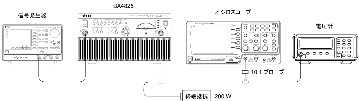
図 6-2 最大出力電圧の測定
