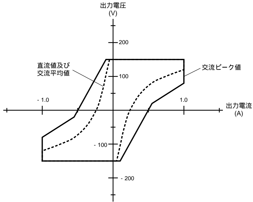
図 4-2 動作領域 (±150 V レンジ)
