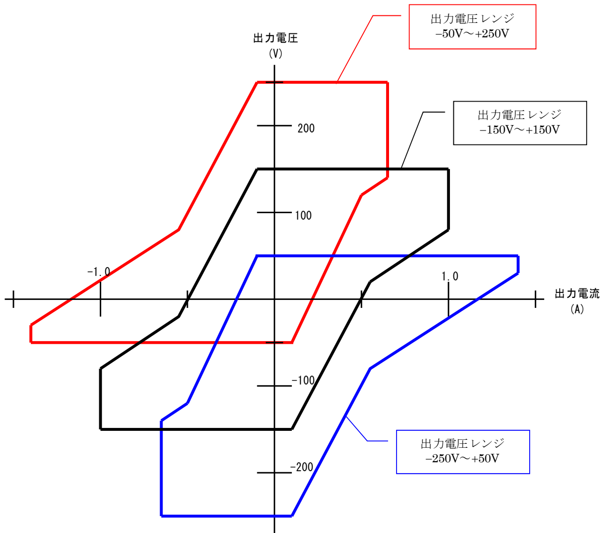
図 7-1 出力電圧・電流範囲 (AC)
