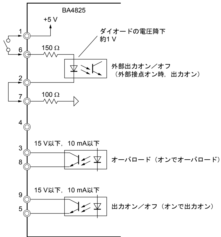
図 3-3 外部制御入出力
