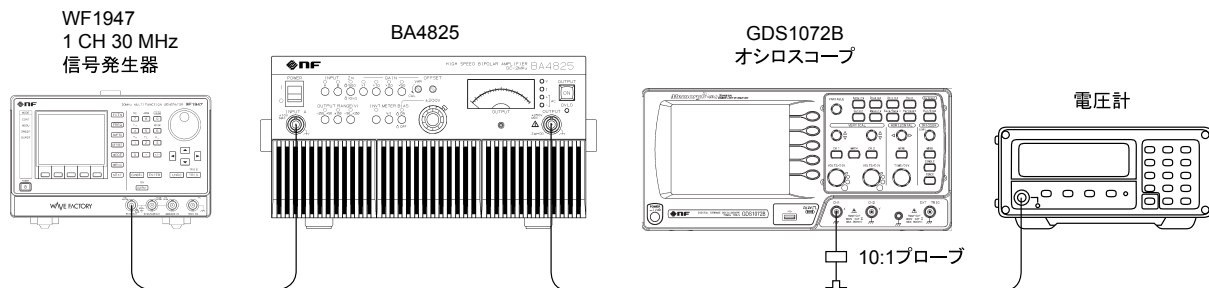
図 2-1 標準的な接続図
