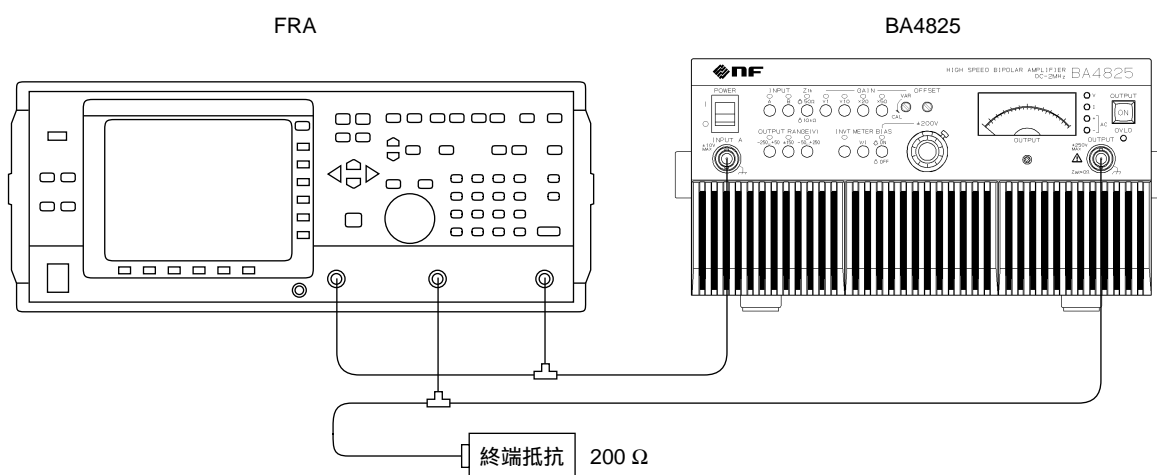
図 6-4 周波数特性の測定
